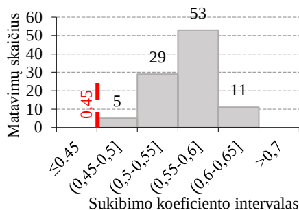
E.1 pav. Skaitinės charakteristikos sukibimo koeficiento paviršiaus apdaro dangos D_{(IV)} užpildo kelio Nr. 3404, matavimo 1
