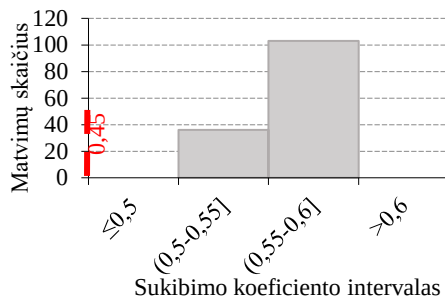
E.1 pav. Skaitinės charakteristikos sukibimo koeficiento paviršiaus apdaro dangos D_{(IV)} užpildo kelio Nr. 3404, matavimo 1
