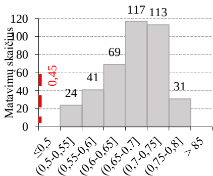
E.2 pav. Skaitinės charakteristikos sukibimo koeficiento paviršiaus apdaro dangos D_{(IV)} užpildo kelio Nr. 3404, matavimo 2
