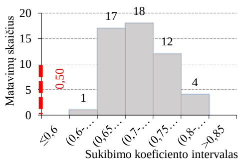
E.9 pav. Skaitinės charakteristikos sukibimo koeficiento AC 11 VS dangos D_{(IV)} užpildo kelio Nr. A4 ruožo 2
