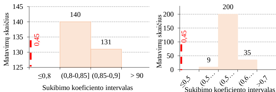
E.5 pav. Skaitinės charakteristikos sukibimo koeficiento paviršiaus apdaro dangos G_{(IV)} užpildo kelio Nr.5202 ruožo
