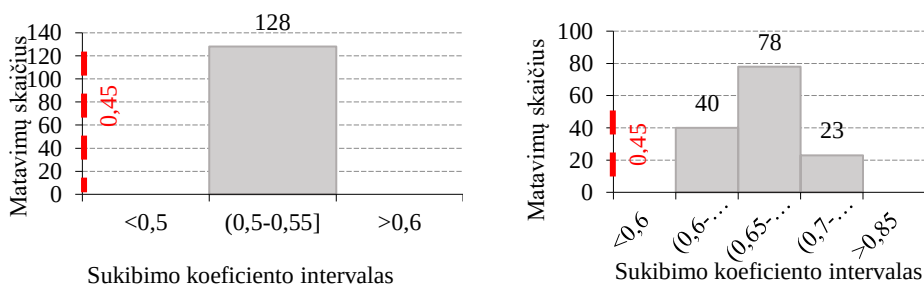
E.7 pav. Skaitinės charakteristikos sukibimo koeficiento AC 11 VS dangos D_{(IV)} užpildo kelio Nr.136 ruožo 1
