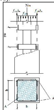
3. pav. Mūro sustiprinto plieninių kampuočių apvaskalu, skaičiuotinė schema
