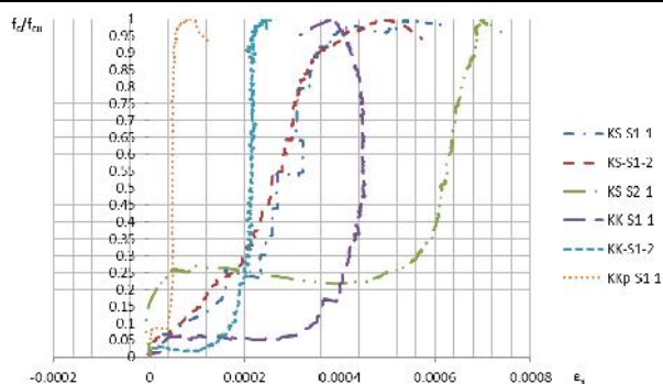
9. pav. Kampuočių vertikaliosios deformacijos priklausomybė nuo santykinio mūro įtempio
