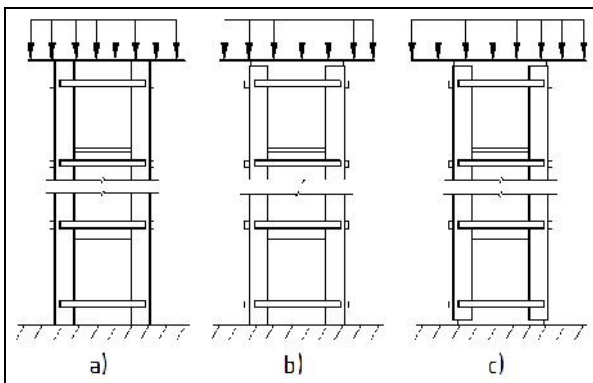
2. pav. Plieninio apvaskalo apkrovimo ir atrėmimo tipai. a – apvaskalas atrėmtas ir tiesiogiai apkrautas apkrova; b – apvaskalas atrėmtas, bet tiesiogiai neapkrautas apkrova; c – apvaskalas neatrėmtas ir tiesiogiai neapkrautas apkrova.
