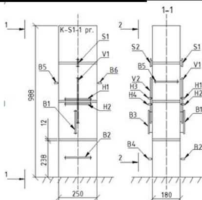
7. pav. Deformacijų matavimo prietaisų ant kontrolinių bandinių išdėstymo schema
