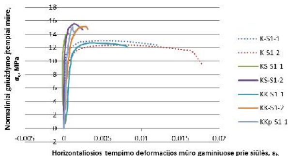
Pav. 10. Bandinių su S1 skiediniu horizontalių deformacijų ir normalinių mūro įtempių priklausomybės
