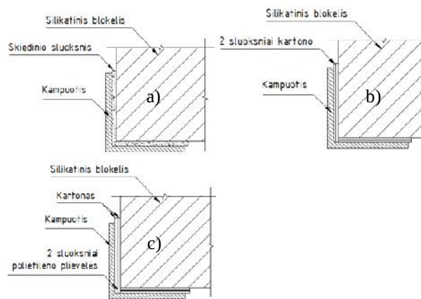
6. pav. Tarpinių sluoksnių įrengimo schemas; a - kampuočiai glaudžiamas per skiedinio sluoksnį; b - kampuočiai glaudžiamas per du kartono sluoksnius; c - kampuočiai glaudžiamas per du kartono sluoksnius su polietileno intarpu
