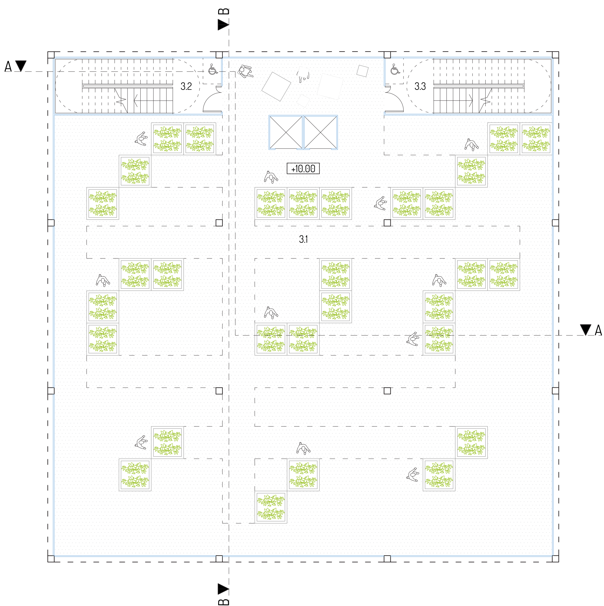
tipinio aukšto planas m 1:100
