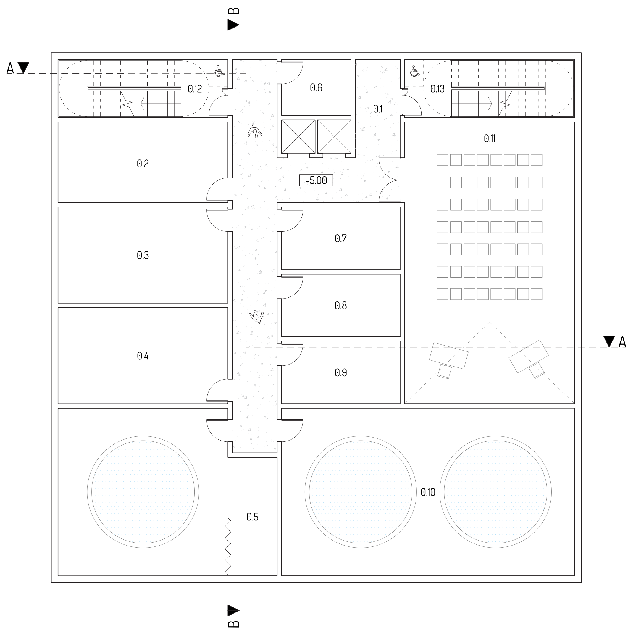
požeminio aukšto planas m 1:100
