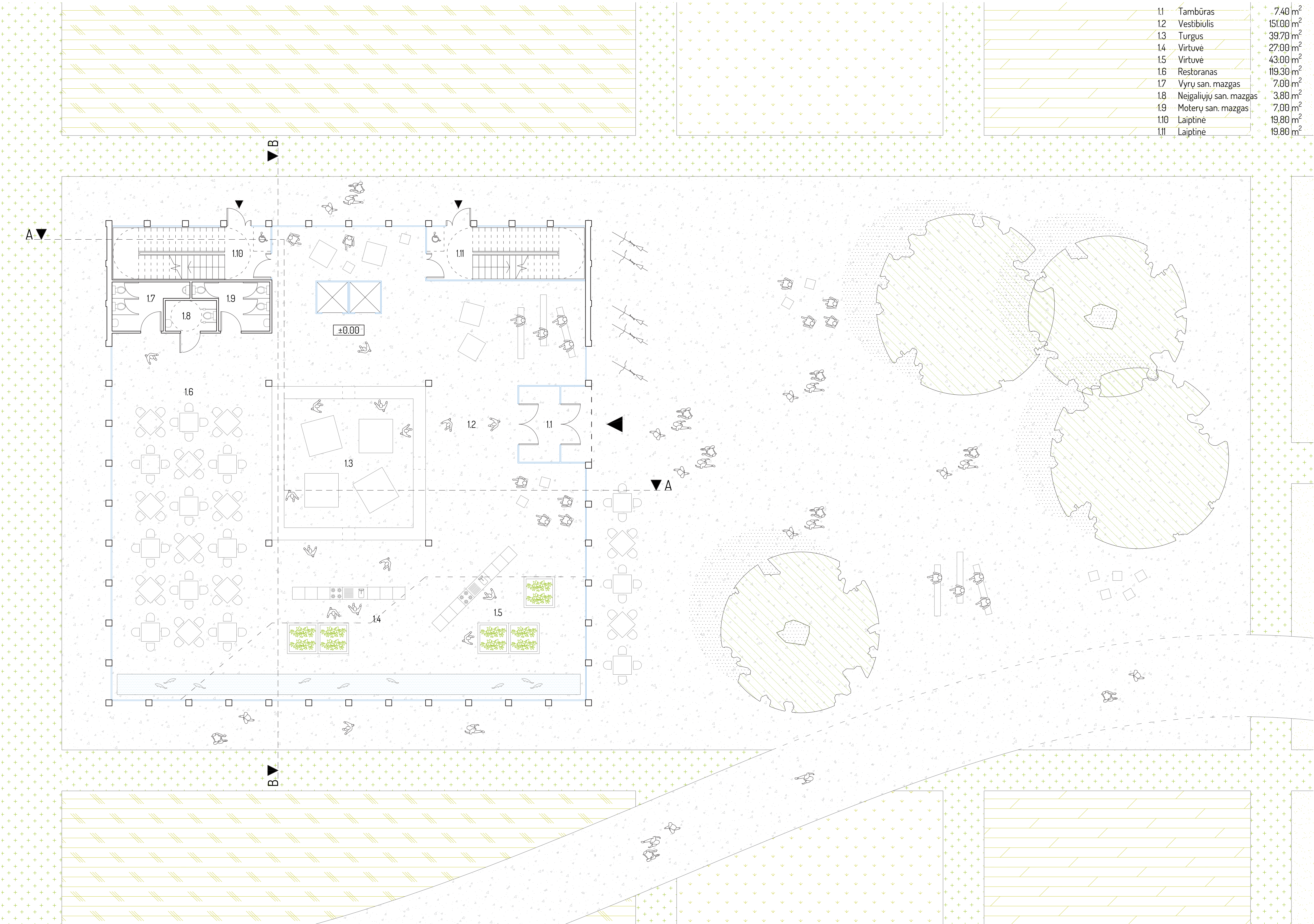
pirmo aukšto planas m 1:100
