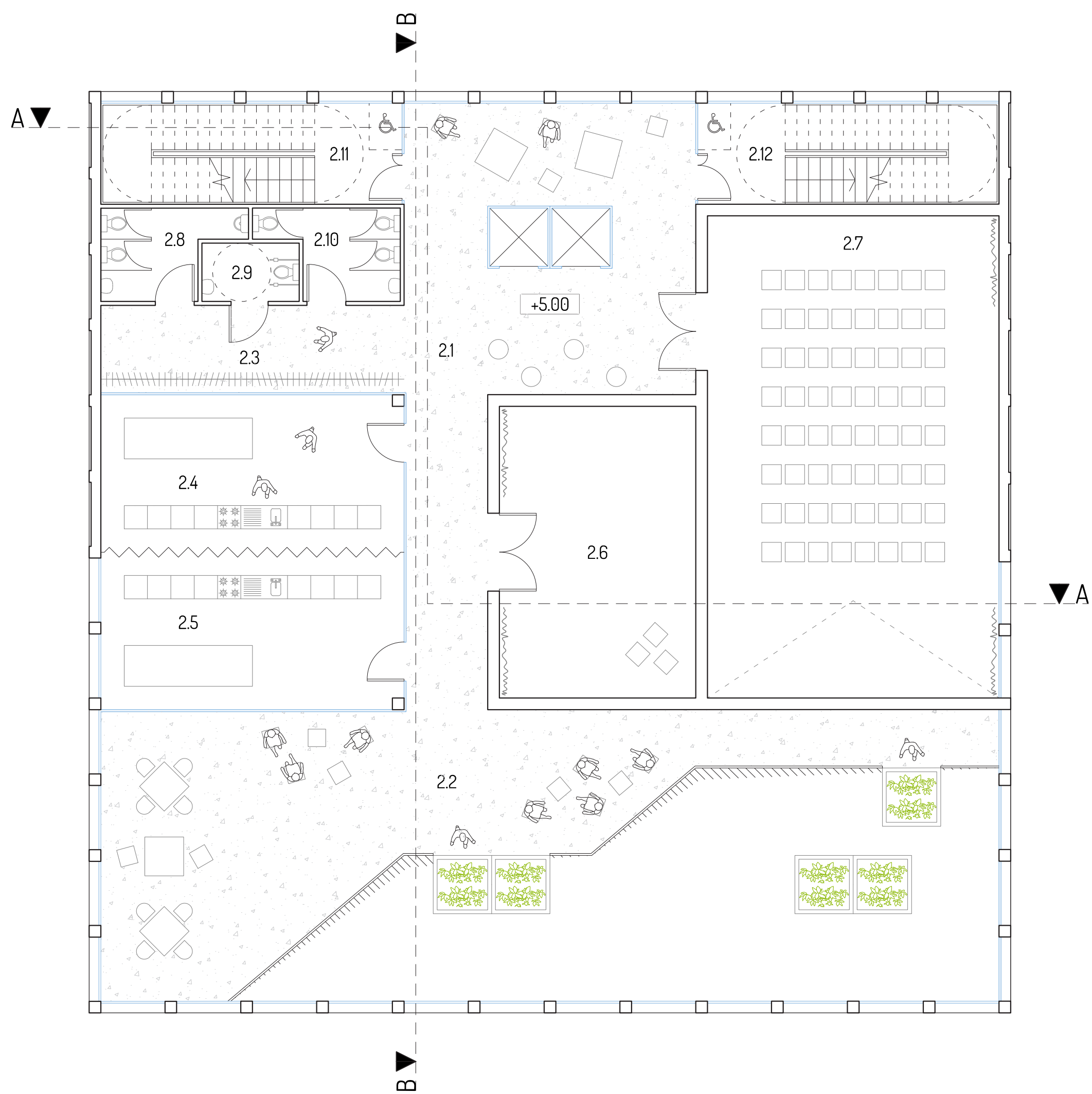
antro aukšto planas m 1:100
