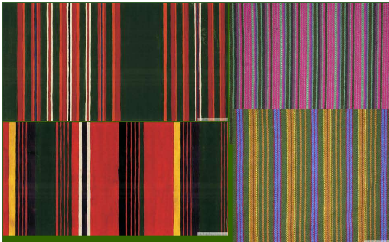
45 pav. Sijono audiniai. Rekonstrukcijos pagal PՅՄ ԴՄՅ 8762, než. viet.; pagal LNM, Tauragės r., Batačiai; pagal LNM S 4214, Mažeikiai; pagal LNM, Plungės r., Alsėdžių apyl.
