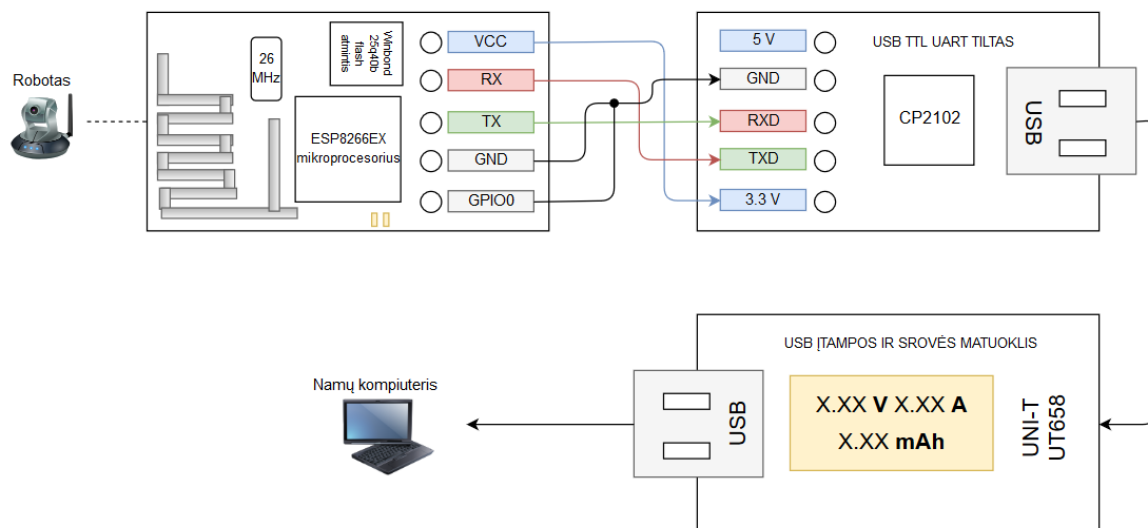
3.7 pav. Kompiuterio USB, ESP8266, tilto ir matuoklio sujungimo schema
