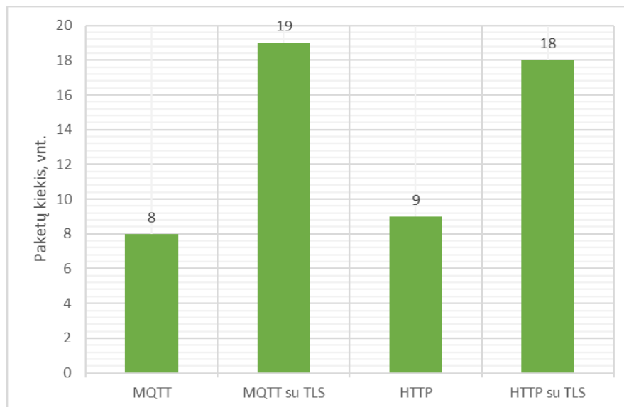
4.13 pav. Komunikacijai reikalingas paketų kiekis
