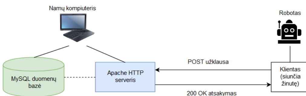
3.2 pav. HTTP serverio – kliento architektūros funkcinė schema
