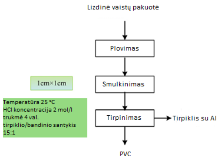
1.10. pav. Lizdinės vaistų pakuotės skyrimo HCl reagentu proceso schema [43]
