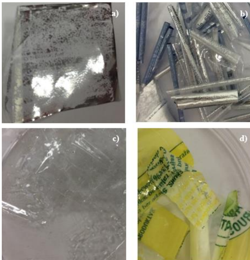
3.7. pav. Aliuminiu dengtos plėvelės pakuotės pokyčiai po skyrimo: a) pakuotės pokyčiai po skyrimo rūgštimi; b) pakuotės pokyčiai po skyrimo organiniu tirpikliu; c) atsiskyrusi pakuotės dalis po skyrimo rūgštimi; d) atsiskyrusi pakuotės dalis su dažais po skyrimo rūgštimi
