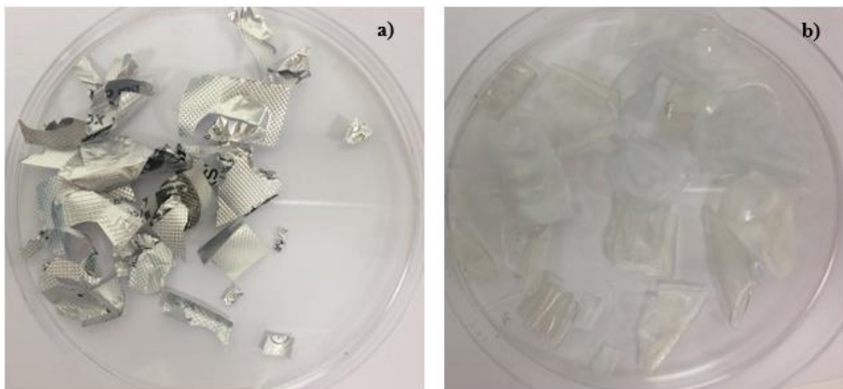
3.6. pav. Lizdinės vaistų pakuotės skyrimo mišriu organiniu tirpikliu rezultatai: a) aliuminio folijos sluoksnis, b) polivinilchlorido sluoksnis
