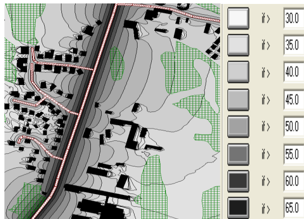
6 pav. Bendra triukšmo sklaida pietinėje miesto dalyje L_{dvn} Fig. 6. General noise dispersion in the southern part of the city L_{den}
