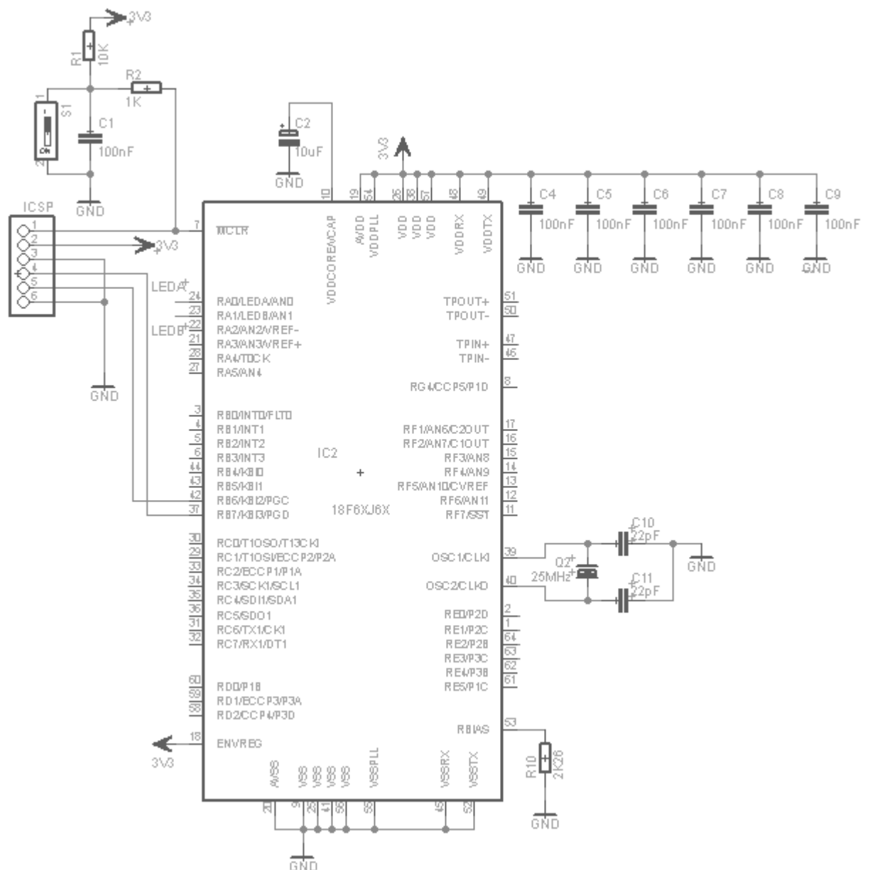
5.1 pav. Mikrovaldiklio grandinė
