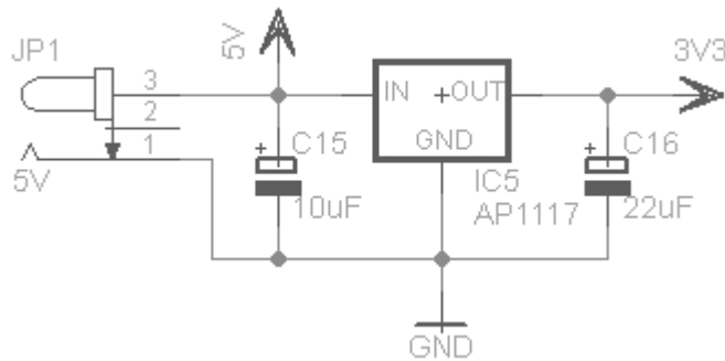
5.3 pav. Maitinimo grandinė
