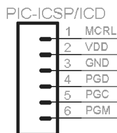
5.2 pav. ICSP jungtis
