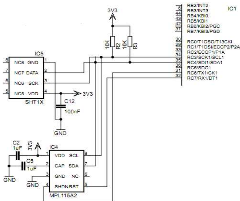
5.5 pav. Jutiklių grandinė
