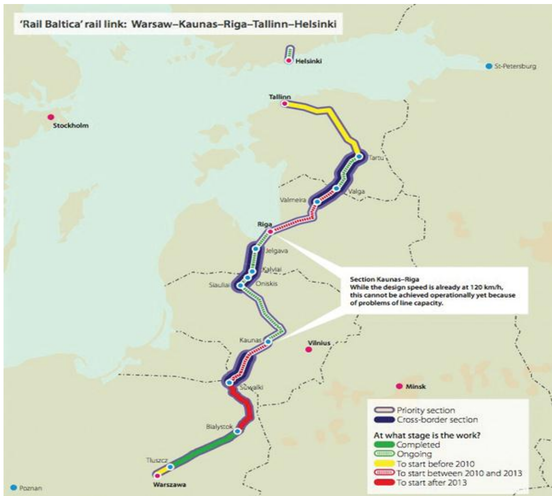
7 pav. „Rail Baltica“ geležinkelio linija (šaltinis: http://www.railwaypro.com/wp/?p=8094 , 2012 – 02 – 24)
