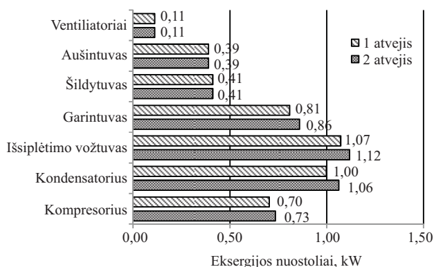
8 pav. Vidutinių eksergijos nuostolių sistemos komponentuose pasiskirstymas
