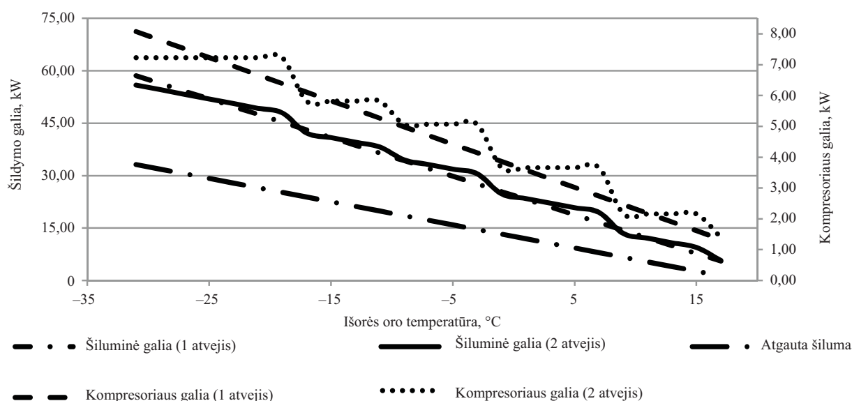
4 pav. Atgautas šilumos kiekis ir kompresorių galios esant įvairioms lauko oro temperatūroms
