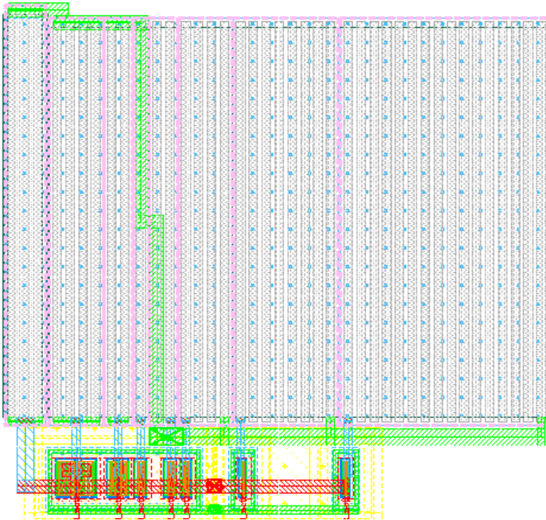
A.1 pav. 6 k \Omega nominalo LRM topologija. Užimamas plotas: 32 \mu\text{m} \times 31,2 \mu\text{m}
