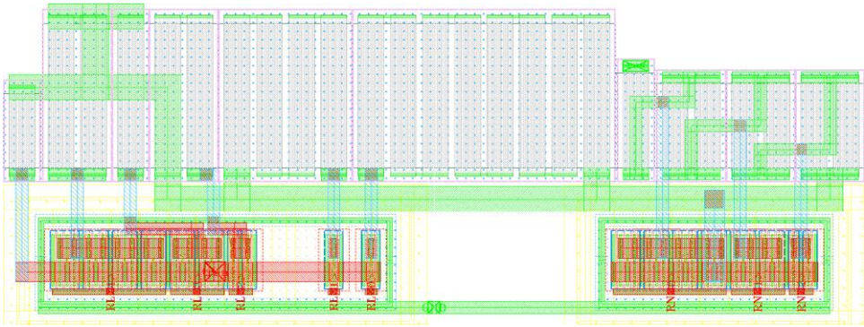
A.2 pav. 6 k \Omega nominalo NLRM topologija. Užimamas plotas: 33,4 \mu\text{m} \times 12,5 \mu\text{m}
