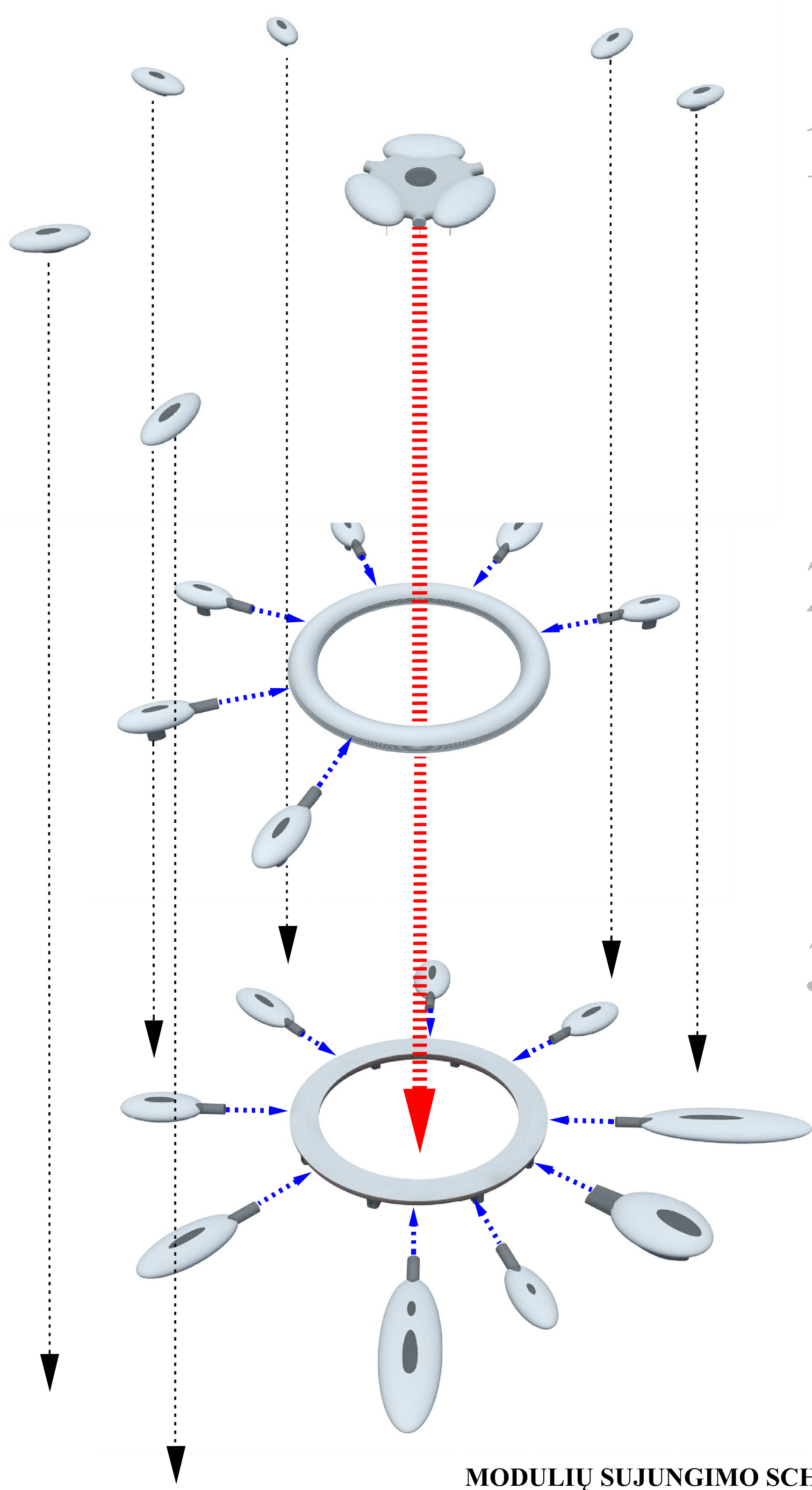
MODULIŲ SUJUNGIMO SCHEMA
