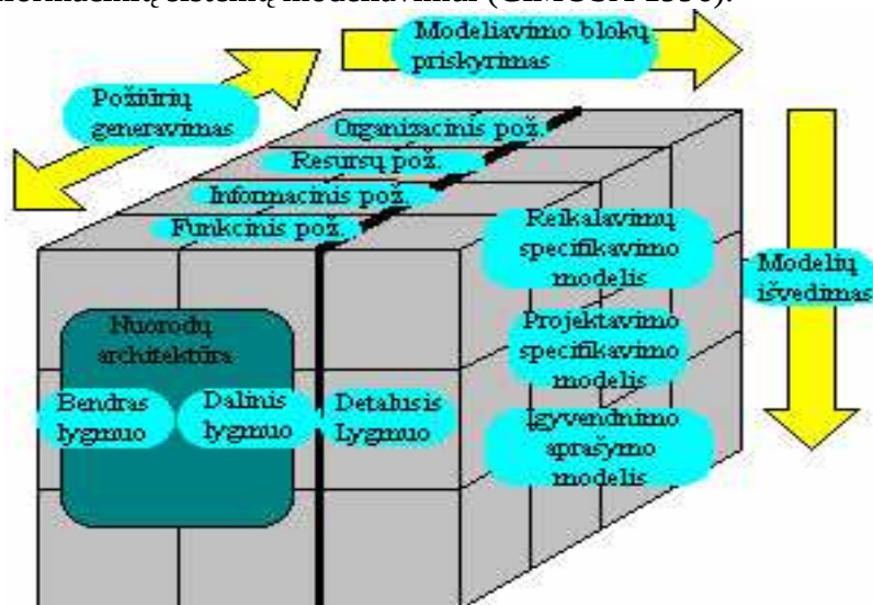
6 Pav. CIMOSA standarto principinė modeliavimo schema
