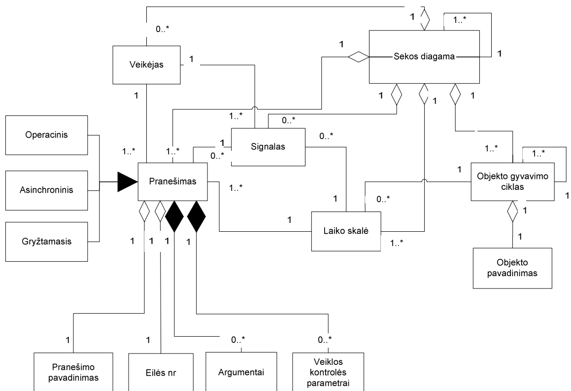
4pav. UML sekų metamodelis
