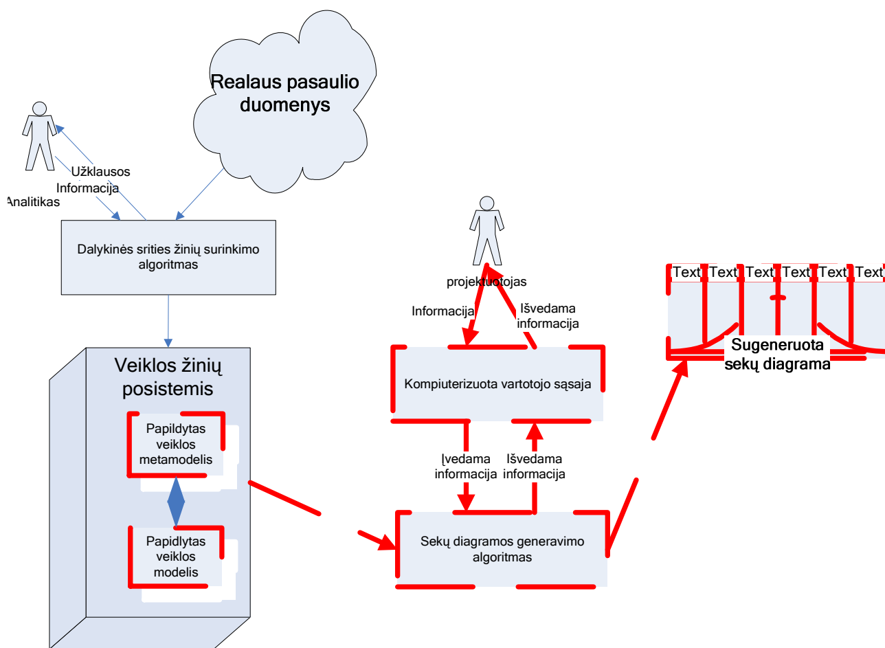
14 pav. Sekų modelio generavimo iš veiklos modelio principinė schema
