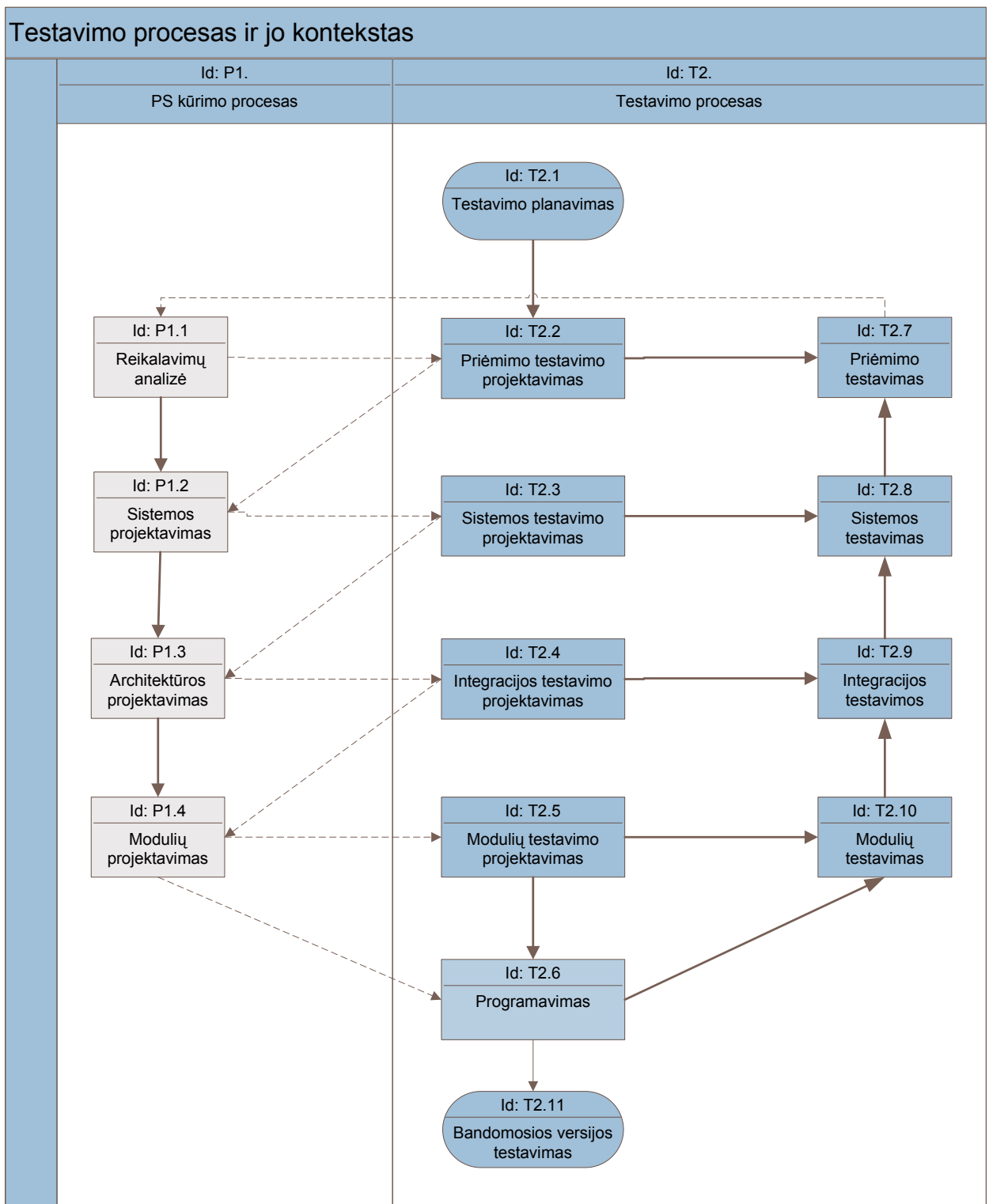
8 pav. Siūlomas programų sistemų testavimo modelis.
