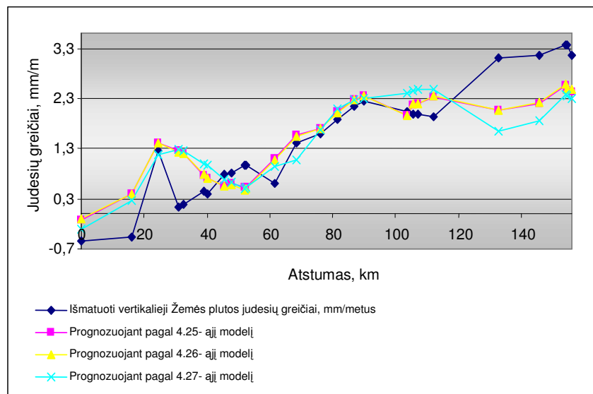
B8 PRIEDAS. Išmatuotų ir prognozuotų vertikaliųjų Žemės plutos judesių 3 poligone linijoje Jonava–Zarasai–Turmantas grafikas
