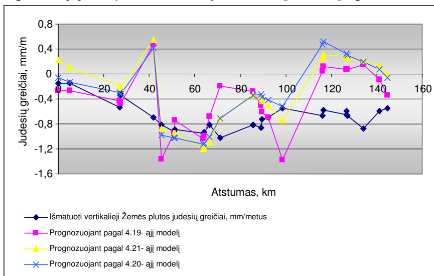
B1 PRIEDAS. Išmatuotų ir prognozuotų vertikaliųjų Žemės plutos judesių 1 poligone linijoje Mikytai–Šilutė–Klaipėda–Palanga–Būtingė grafikas
