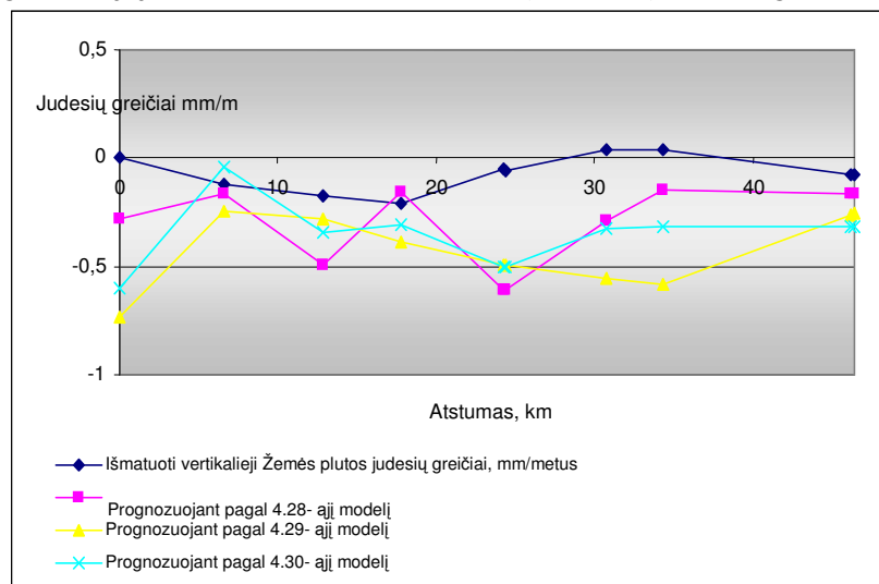
B12 PRIEDAS. Išmatuotų ir prognozuotų vertikalųjų Žemės plutos judesių 5 poligone linijoje Vilnius–Baranovičiai grafikas
