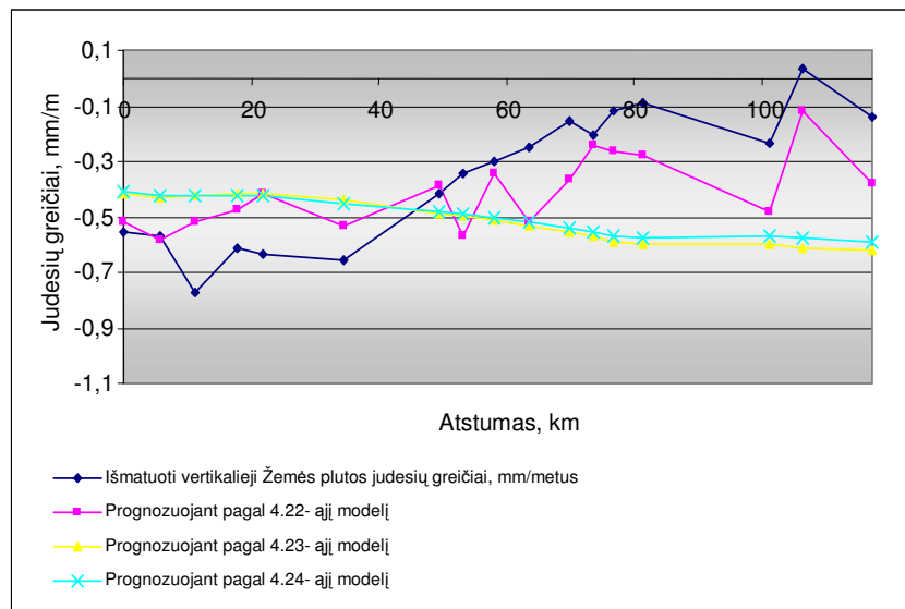
B6 PRIEDAS. Išmatuotų ir prognozuotų vertikalųjų Žemės plutos judesių 2 poligone linijoje Jonava–Šiauliai grafikas
