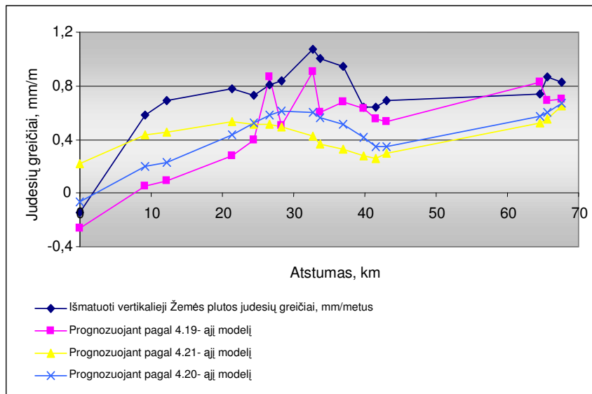
B3 PRIEDAS. Išmatuotų ir prognozuotų vertikalųjų Žemės plutos judesių 1 poligone linijoje Šiauliai–Kūžiai–Mažeikiai–Lūšė grafikas
