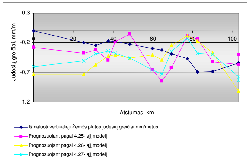
B9 PRIEDAS. Išmatuotų ir prognozuotų vertikaliųjų Žemės plutos judesių 3 poligone linijoje Vilnius–Jonava–Jelgava grafikas
