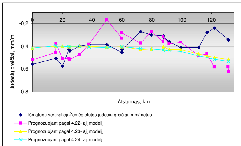
B3 PRIEDAS. Išmatuotų ir prognozuotų vertikalųjų Žemės plutos judesių 1 poligone linijoje Šiauliai–Kūžiai–Mažeikiai–Lūšė grafikas
