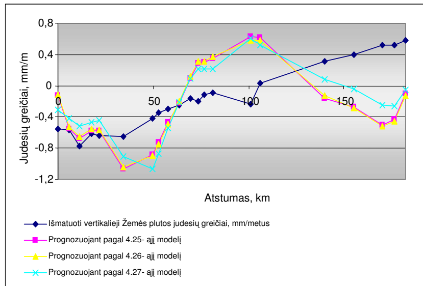
B7 PRIEDAS. Išmatuotų ir prognozuotų vertikaliųjų Žemės plutos judesių 3 poligone linijoje Jonava–Jelgava grafikas
