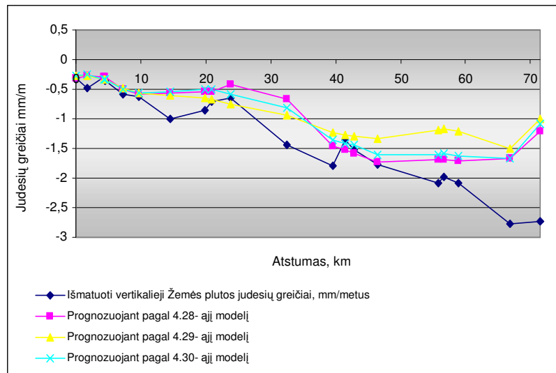
B11 PRIEDAS. Išmatuotų ir prognozuotų vertikalųjų Žemės plutos judesių 5 poligone linijoje Kazlų Rūda–Šeštokai–Lazdijai–Lenkijos siena grafikas
