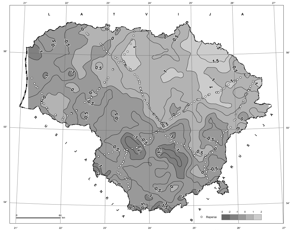
B13 PRIEDAS. Prognostinis dabartinių vertikaliųjų Žemės plutos judesių greičių žemėlapis taikant (4.31) regresinį modelį
