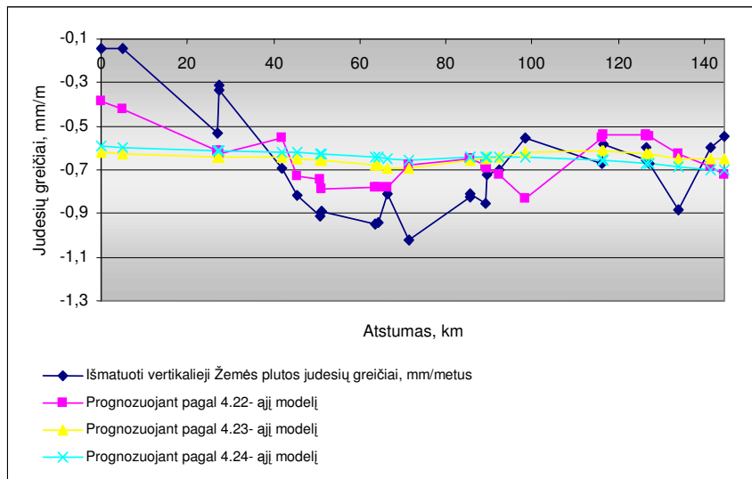
B5 PRIEDAS. Išmatuotų ir prognozuotų vertikalųjų Žemės plutos judesių 2 poligone linijoje Šiauliai–Tauragė–Mikytai grafikas
