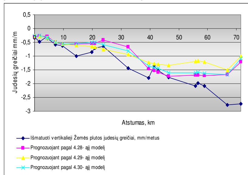
B10 PRIEDAS. Išmatuotų ir prognozuotų vertikaliųjų Žemės plutos judesių 5 poligone linijoje Jonava–Gaižiūnai–Palemonas–Kaunas–Kazlų Rūda–Kybartai grafikas
