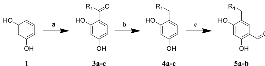
20 pav. Bendra 5-(cikloalkil ar aril)-2,4-dihidroksibenzaldehydų sintezės schema. Reagentai ir sąlygos: (a) karboksirūgštis ( 2a-c , 2 lentelė), BF 3 OEt 2 , 80 °C, 4-5 val.; (b) NaBH 3 CN, HCl, kamb. t., 24 val.; (c) POCl 3 , DMF, kamb. t., 24 val; 50 °C, 4 val.; NaOH, 70 °C, 20 min.
