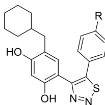
19 pav. Bendra susintetintų junginių su tiadiazolo fragmentu struktūra.
