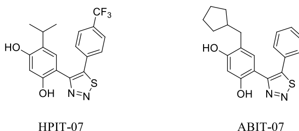
2 pav. 4-izopropil-6-(5-(4-(trifluorometil)fenil)-1,2,3-tiadiazol-4-il)benzen-1,3-diolis (HPIT-07) ir 4-(ciklopentilmetil)-6-(5-fenil-1,2,3-tiadiazol-4-il)benzen-1,3-diolis (ABIT-07).
