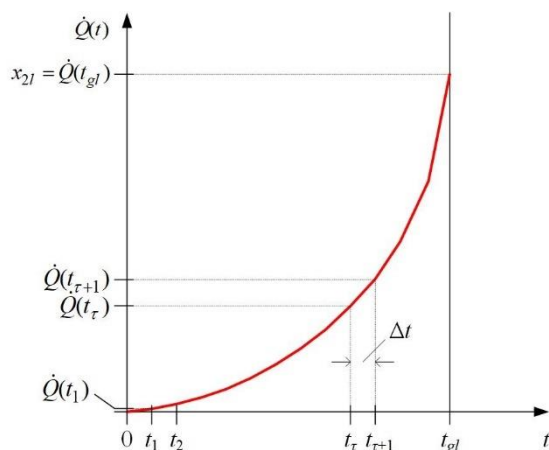
3.7 pav. Gaisro energijos išskyrimo greičio (HRR) proceso modeliavimas
