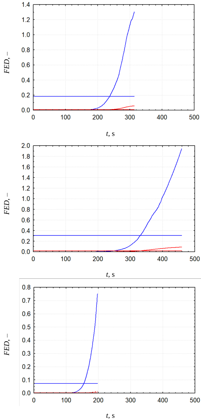
3.11 pav. Dozės FED laiko sekos \{y_{2l}(t_\tau) \equiv FED(t_\tau), l = 1, 25, 50\} ( t_\tau \in [0, t_{gl}] , n_\tau = 1000 ; laiko t_{gl} reikšmės pateiktos A.1 lentelėje; horizontalios linijos rodo laiko sekų vidurkius, pateiktus C priede)
