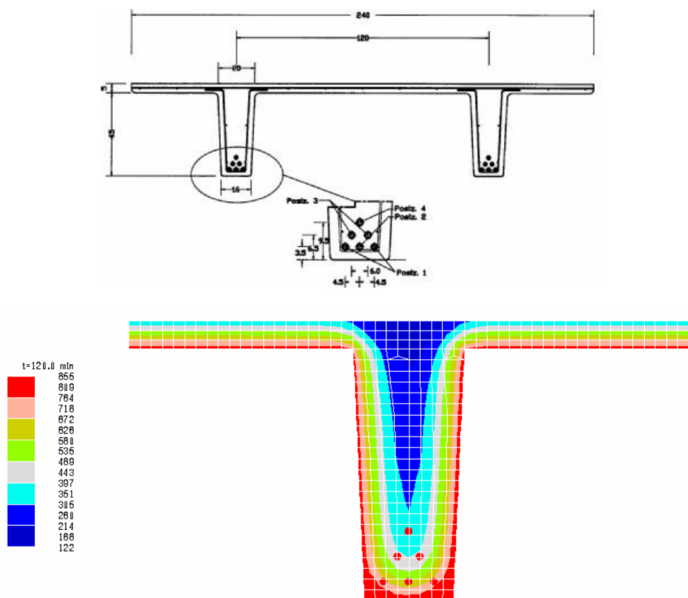
1.4 pav. Temperatūros pasiskirstymo dvigubos T plokštės skerspjūvyje vertinimas, gautas su lauko modelio programa FDS (La Mendola, 2019)
