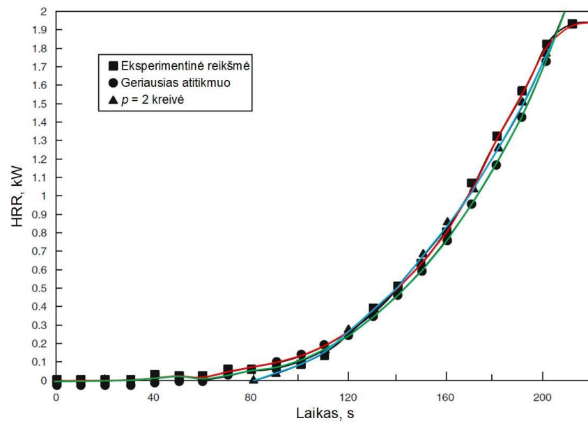
2.5 pav. Empirinė HRR kreivė, gauta deginant kėdę kalorimetre, bei dvi teorinės kreivės, pritaikytos prie empirinių rezultatų (SFPE, 2016)
