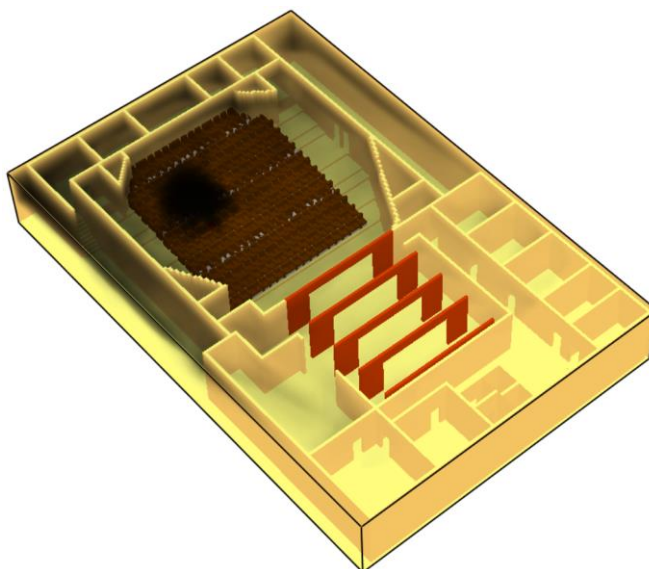
(c) dūmų plitimas, gautas su SMOKEVIEW programa
