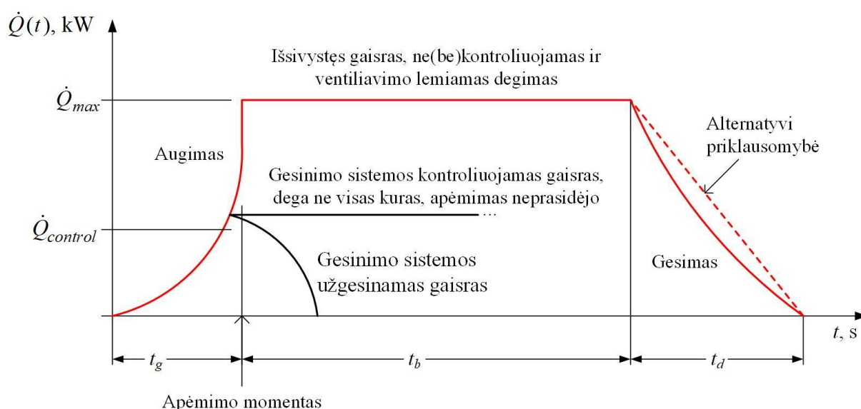
2.4 pav. Gesinimo sistemos įtaka gaisrui, nusakomam projektine gaisro kreive ( \dot{Q}_{control} – HRR reikšmė, kai aktyvuojama gesinimo sistema) (Ingason, 2009; Karlsson & Quintiere, 2000)
