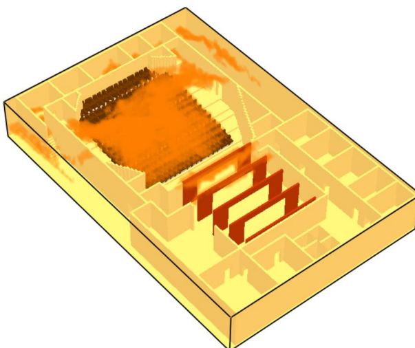
(b) liepsnos plitimas gaisro metu, gautas vizualizuojant su SMOKEVIEW programa
