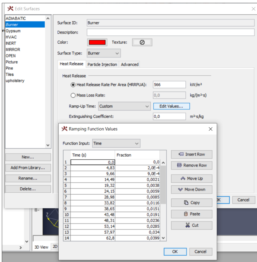
3.8 pav. FDS programos langas, kuriame buvo įvedama maksimali HRRPUA reikšmė x_{2l}/A_{fire} ir HRR kreivę formuojančios reikšmių poros (t_\tau, \dot{Q}(t_\tau)/x_{2l})
