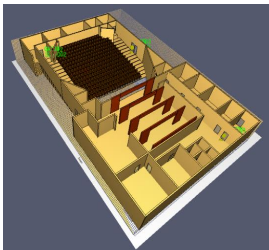
(a) žiūrovų salės modelis, sudarytas FDS programa
