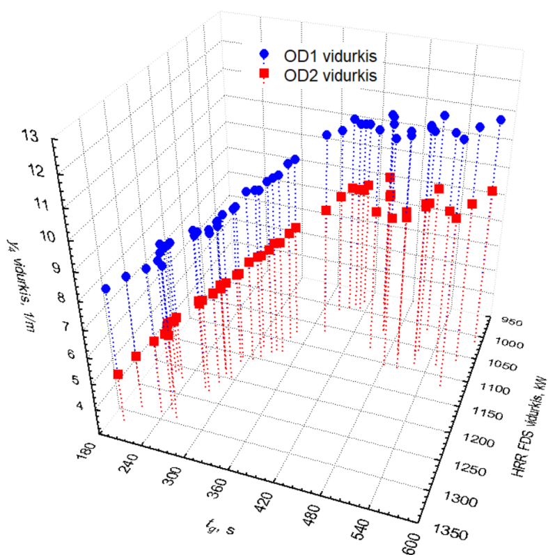
E.1 pav. Taškinės reikšmių trejetų (t_{gl}, \bar{Q}_{FDS,l}, \bar{y}_{3l}) ir (t_{gl}, \bar{Q}_{FDS,l}, \bar{y}_{4l}) ( l = 1, 2, \dots, 50 ) diagramos, susijusios su pirma virtualių matavimo prietaisų vertikale (mėlyni taškai) ir antra virtualių matavimo prietaisų vertikale (raudoni taškai)
