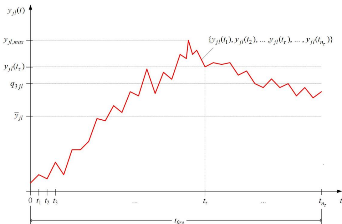
2.9 pav. Grafinė sekos \{y_{jl}(t_1), y_{jl}(t_2), \dots, y_{jl}(t_\tau), \dots, y_{jl}(t_{n_\tau})\} ir jos pagrindu skaičiuojamų dydžių iliustracija
