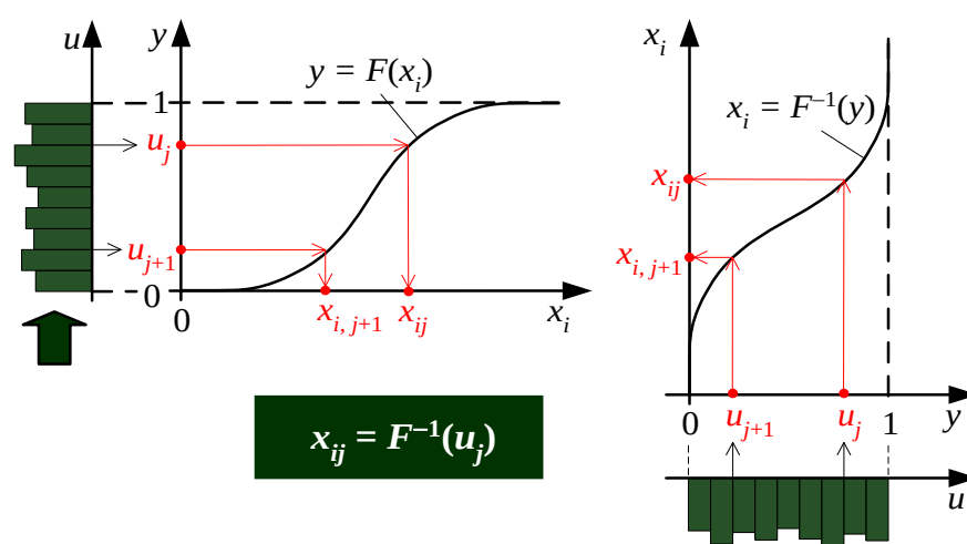
1.6 pav. Atsitiktinio didžio su duotąja pasiskirstymo funkcija F(x) reikšmių generavimo schema, grindžiama atsitiktinių reikšmių U(0, 1) generatoriaus panaudojimu
