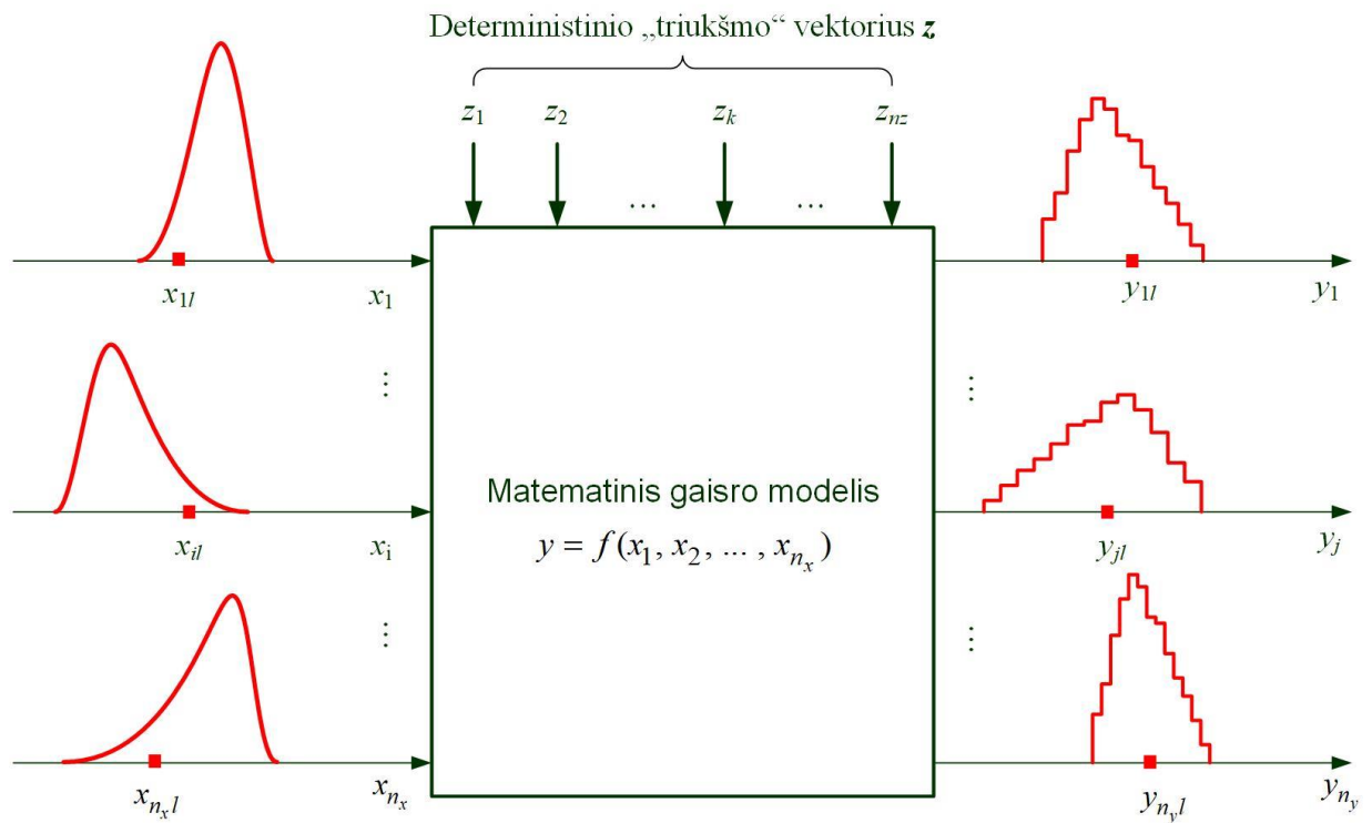
2.1 pav. Gaisro modelio įvesties kintamųjų išskyrimas į atsitiktinius įvesties kintamuosius, išreikštus vektoriumi \mathbf{x} , ir fiksuoto „triukšmo“ kintamuosius, sugrupuotus į vektorių \mathbf{z} (indeksas l nurodo į reikšmę, generuotą modeliavimo cikle su numeriu l (angl. loop ))
