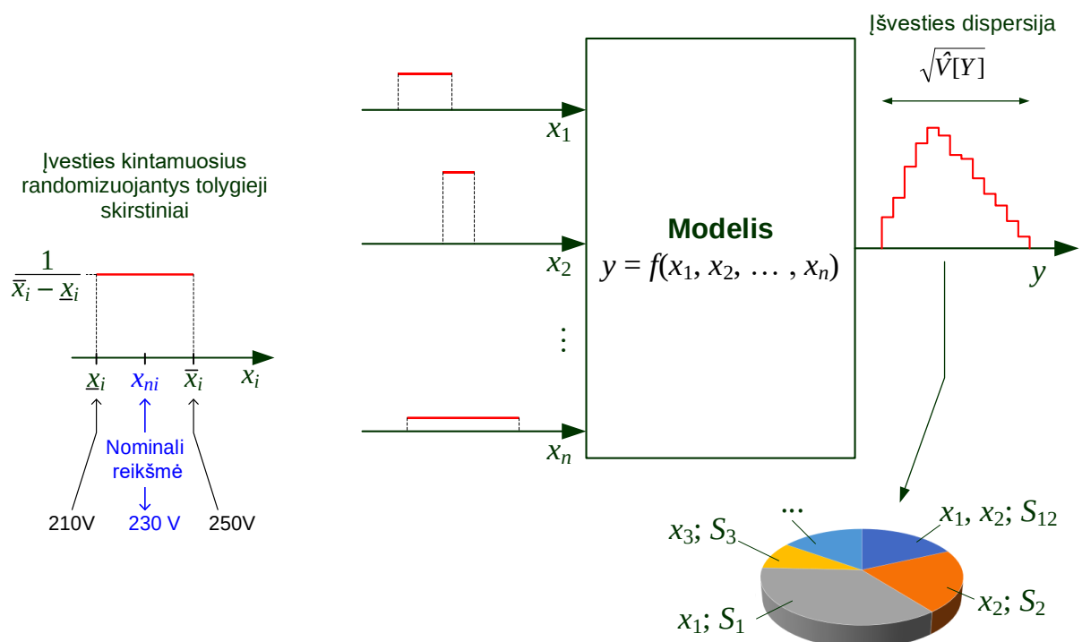
1.10 pav. Įvesties kintamųjų X_i randomizavimas, atliekamas nusakant juos tolygiuoju tikimybių skirstiniu ir taikomas atliekant globaliąją jautrumo analizę
