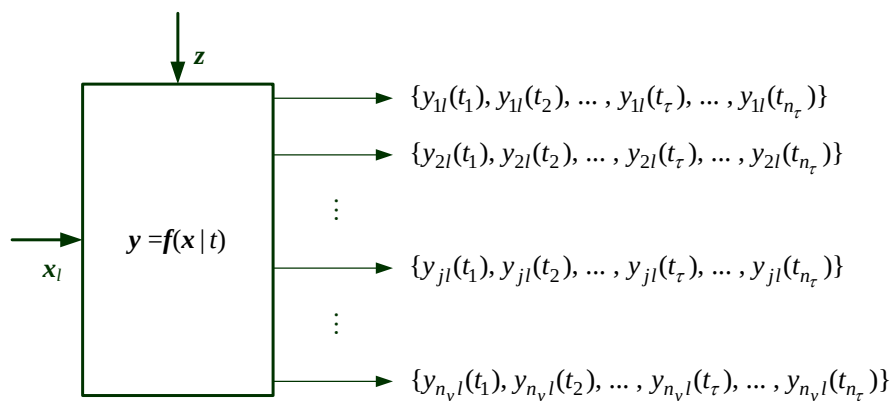
2.8 pav. Modeliavimo ciklo l teikiama informacija, išreikšta gaisro charakteristikų reikšmių sekų \{y_{jl}(t_1), y_{jl}(t_2), \dots, y_{jl}(t_\tau), \dots, y_{jl}(t_{n_\tau})\} pavidalu
