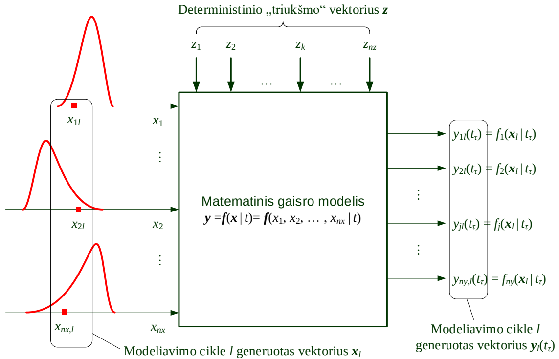
2.7 pav. Grafinė gaisro modeliavimo ciklo l , kuriame apskaičiuojama išvesties kintamųjų vektorių seka \{y_l(t_1), y_l(t_2), \dots, y_l(t_\tau), \dots, y_l(t_{n_\tau})\} , iliustracija, atitinkanti skaičiavimo su modeliu f(\mathbf{x} | t) žingsnį t_\tau
