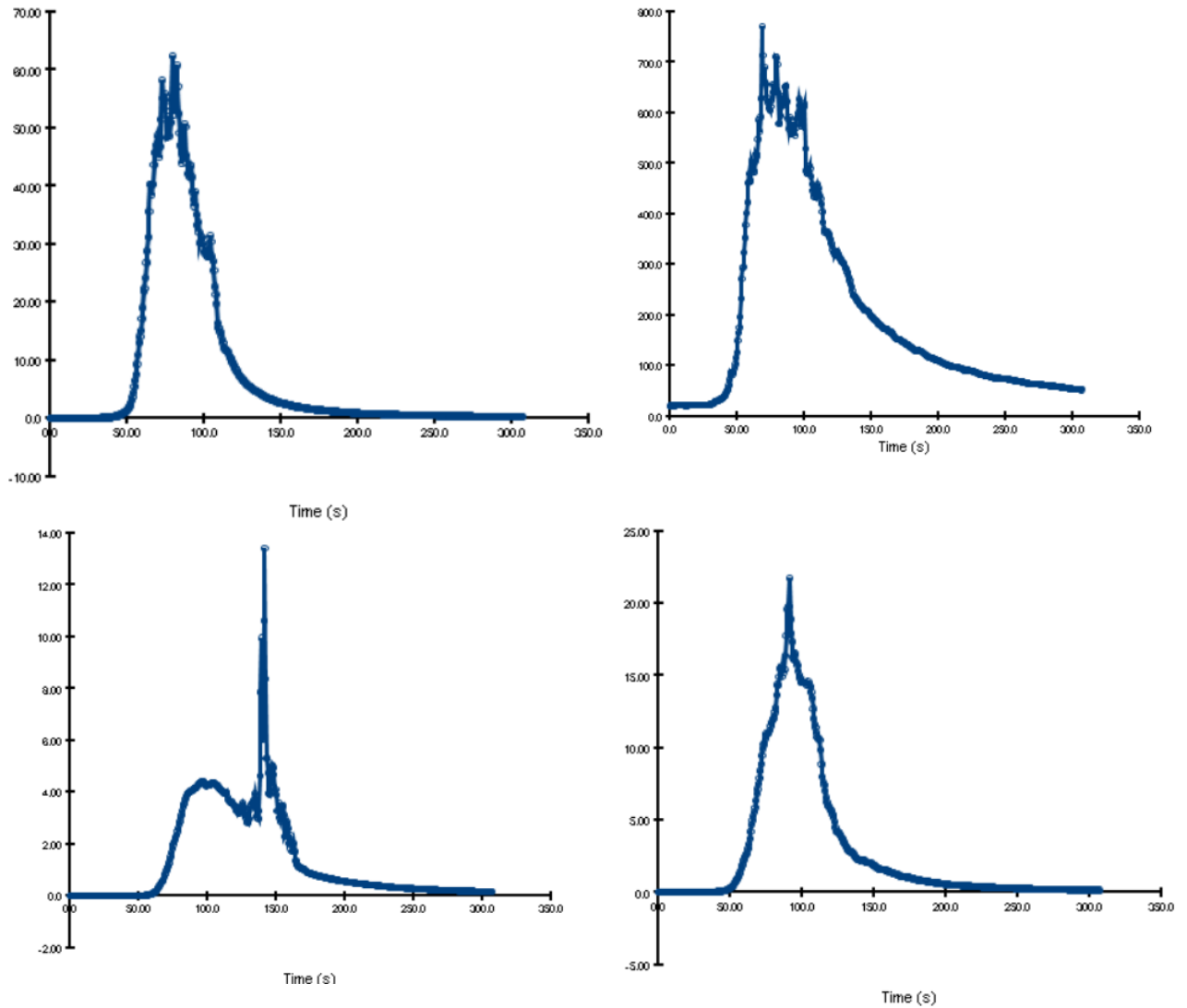
2.12 pav. Keturios šiluminės spinduliuotės laiko sekos, apskaičiuotos užprogramavus virtualius radiometrus, naudotomis modeliuojant žiūrovų salės gaisrą (vertikalios ašies dimensija visur yra \text{kW/m}^2 )
