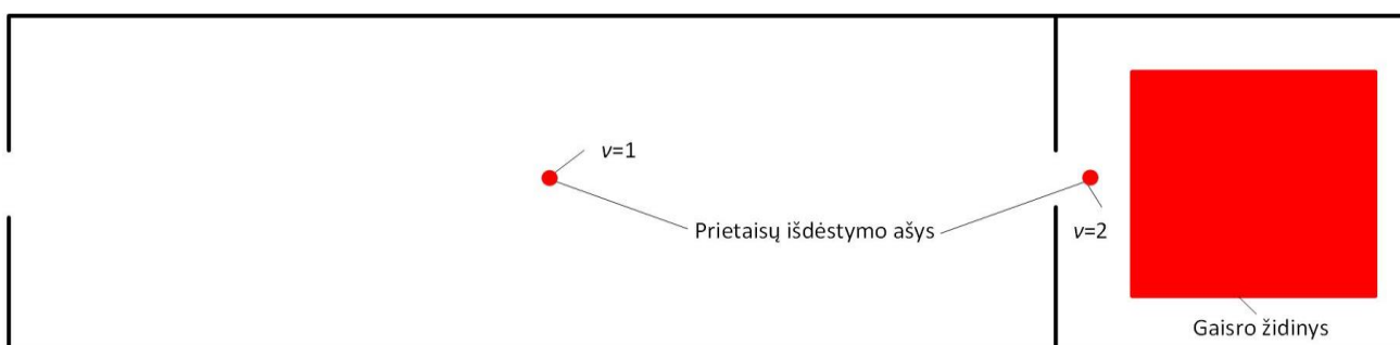
3.3 pav. Schema, vaizduojanti keturias gaisro kilimo vietas bei tris grupes vertikaliai išdėstytų prietaisų (jutiklių), kuriais gaisro modeliavimo metu buvo matuojami su žmonių sauga susiję gaisro poveikiai
