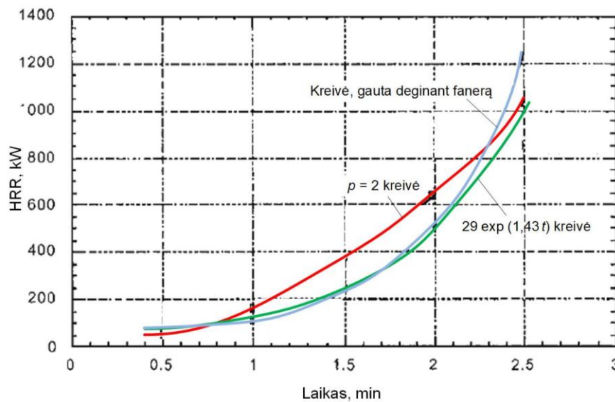
2.6 pav. Faneros bandymo kalorimetre HRR rezultatai bei kvadratinė ir eksponentinė kreivės pritaikytos prie šių rezultatų (Högländer & Sundström, 1997)
