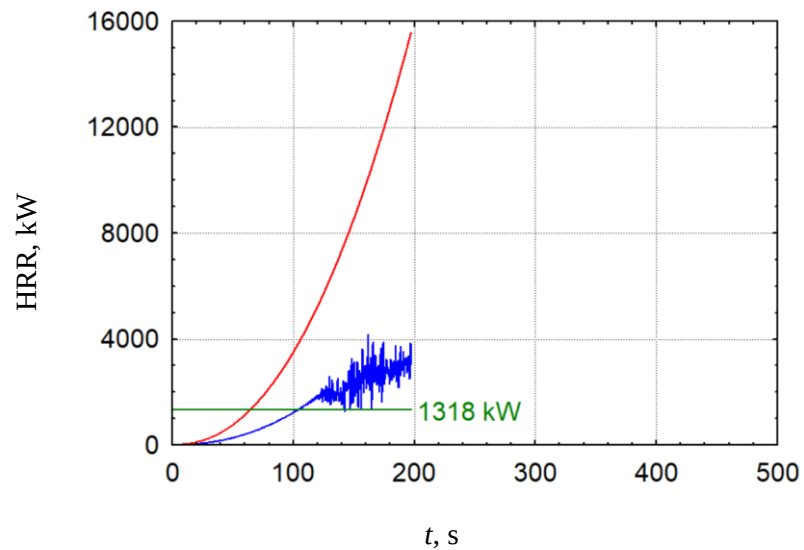
3.13 pav. Parinktosios HRR funkcijos \dot{Q}(t_\tau) ir FDS programos generuotos HRR funkcijos laiko sekų grafikai, išreikšti, atitinkamai, monotoniškai kylančia kreive ir osciliuojančia kreive ir sudaryti stochastinio modeliavimo ciklams l = 1, 25, 50 ( n_\tau = 1000 ) (horizontalios linijos yra HRR reikšmių vidurkiai)
