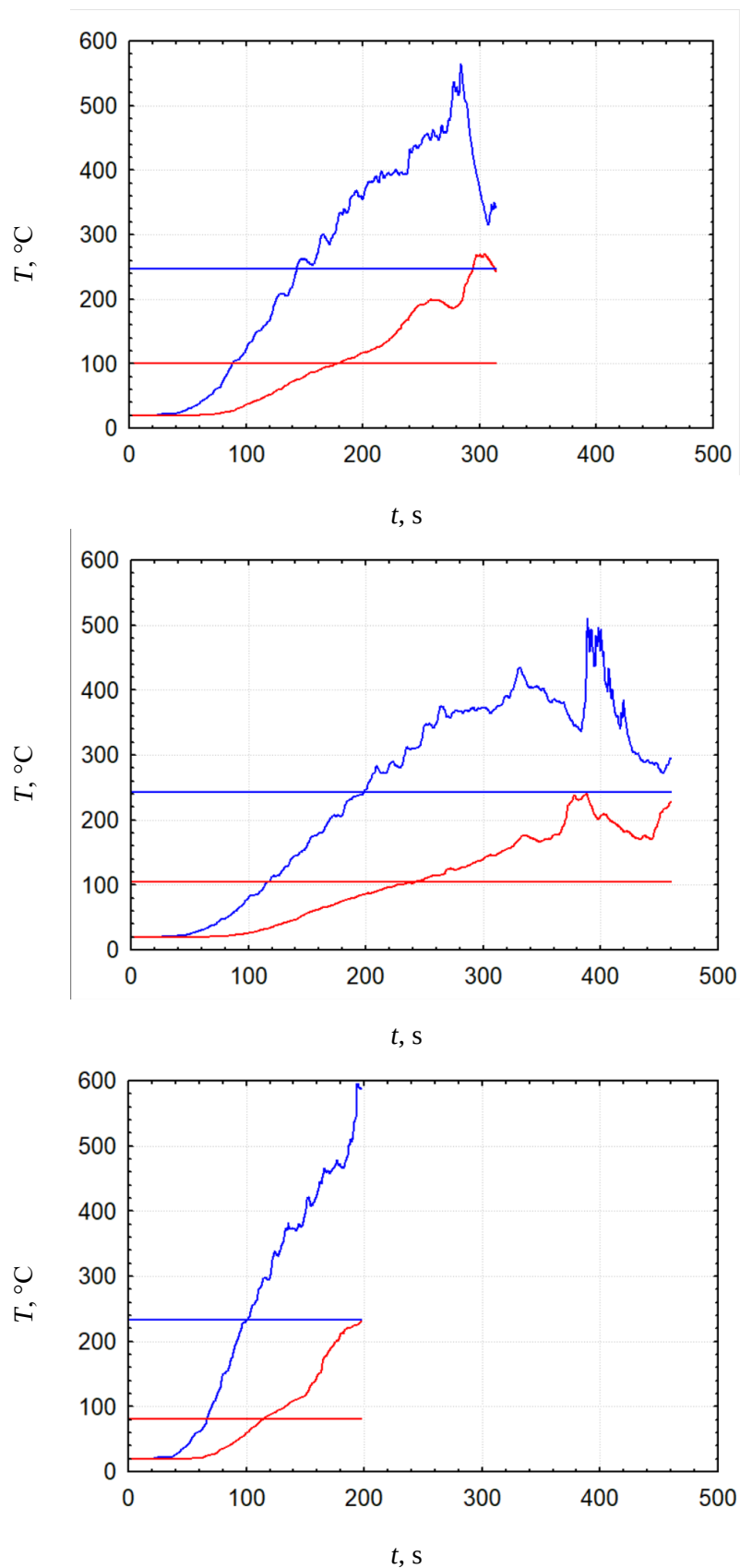
3.9 pav. Temperatūros laiko sekos \{y_{ll}(t_\tau) \equiv T(t_\tau), l=1, 25, 50\} ( t_\tau \in [0, t_{gl}] , n_\tau = 1000 ; laiko t_{gl} reikšmės pateiktos A.1 lentelėje; horizontalios linijos rodo laiko sekų vidurkius, pateiktus C priede)
