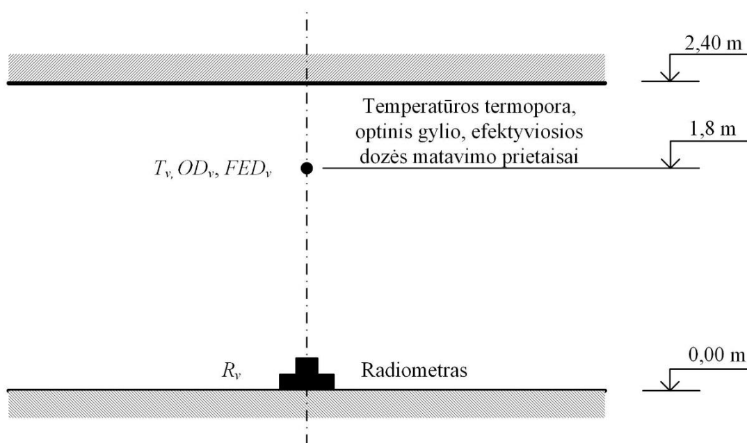
3.4 pav. Virtualių gaisro charakteristikų matavimo prietaisų (jutiklių) išdėstymo schema vertikalyje, kurios numeris yra v ( v = 1, 2 ), kurie fiksuoja gaisro charakteristikas
