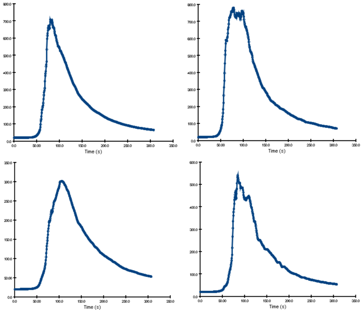
2.11 pav. Keturios temperatūros laiko sekos, užfiksuotos virtualiomis termoporomis, naudotomis modeliuojant žiūrovų salės gaisrą (vertikaliosios ašies dimensija visur yra °C)
