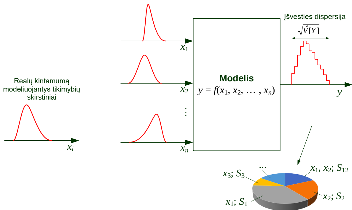
1.9 pav. Globalioji jautrumo analizė įvesties kintamuosius X_i modeliuojant tikimybių skirstiniais
