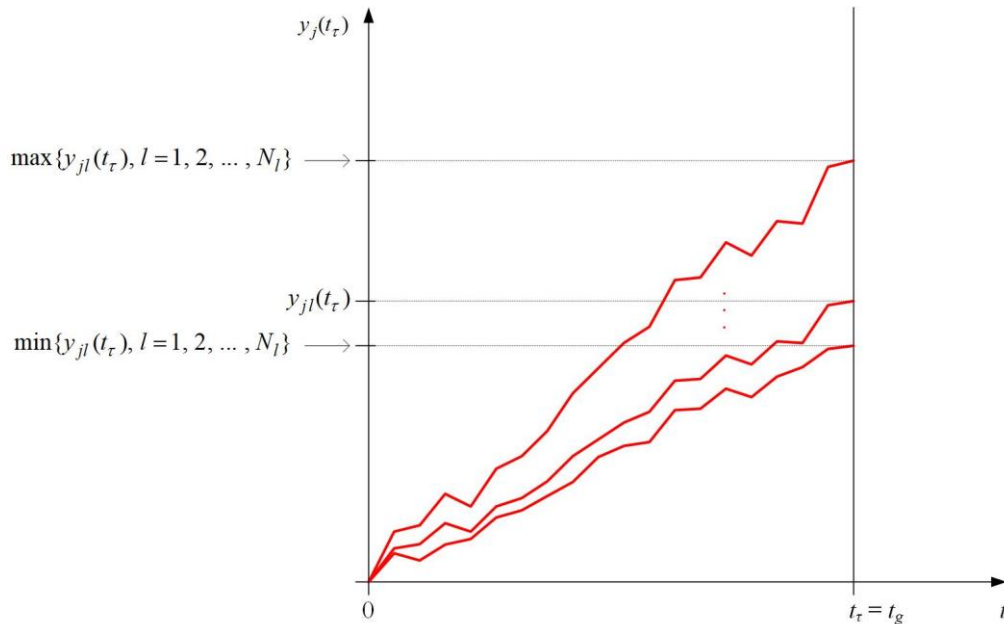
2.14 pav. Schema, vaizduojanti išvesties kintamojo y_j reikšmių sekas, gautas stochastiškai modeliuojant, baigiamas laiko momentu t_\tau ir naudojamas sudaryti šio kintamojo reikšmių aibę \{y_{jl}(t_\tau), l=1, 2, \dots, N_l\} , skirtą jautrumo analizei
