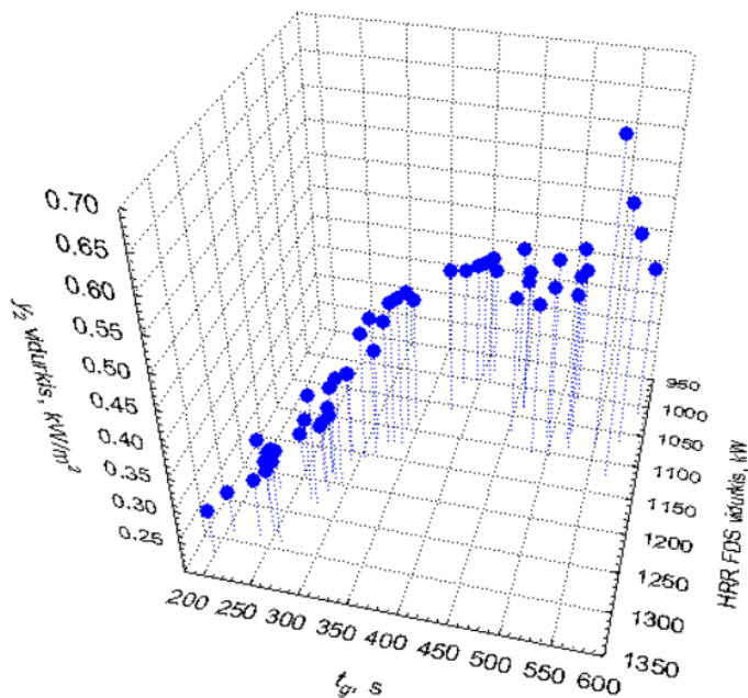
3.14 pav. Taškinės reikšmių trejetų (t_{gl}, \bar{\bar{Q}}_{FDS,l}, \bar{y}_{1l}) ir (t_{gl}, \bar{\bar{Q}}_{FDS,l}, \bar{y}_{2l}) ( l = 1, 2, \dots, 50 ) diagramos, atskleidžiančios augimo ciklo trukmės laiko t_g dydžių įtaką \bar{y}_{1l} , \bar{y}_{2l} ir \bar{\bar{Q}}_{FDS,l} priklausomybėms
