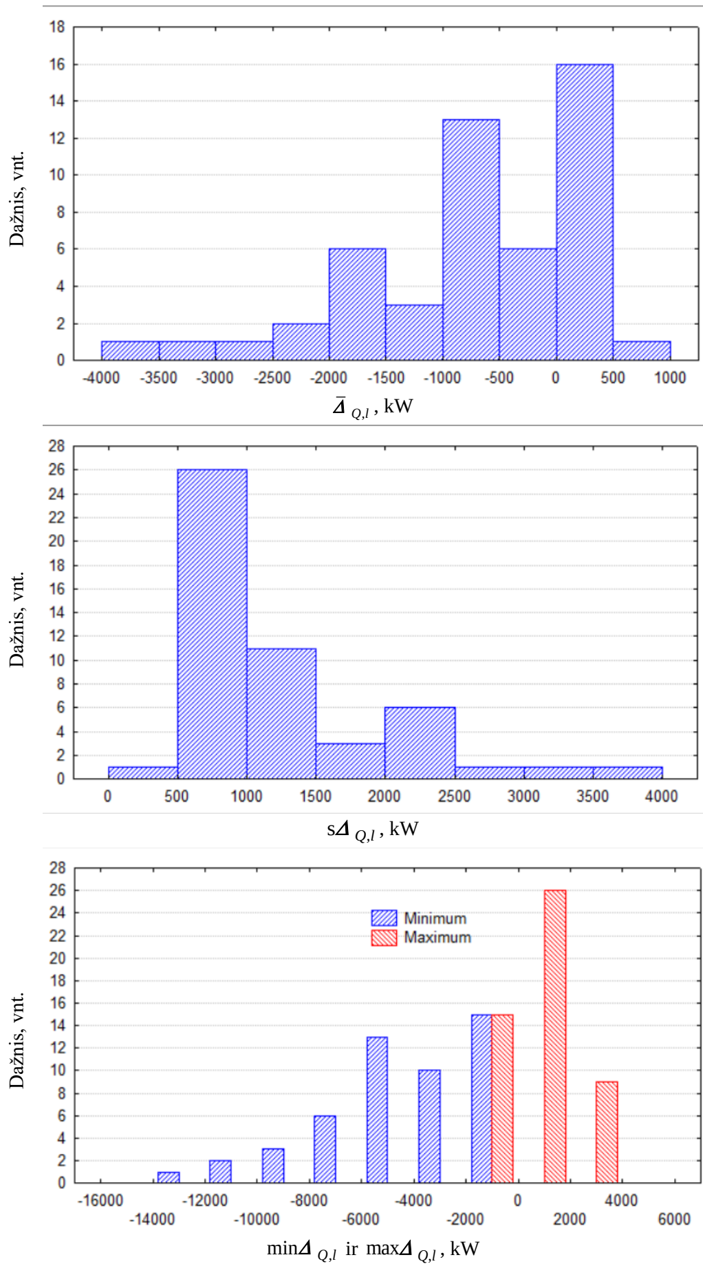
3.16 pav. Histogramos, sudarytos imčių \Delta_{Q,l} = \{\dot{Q}_l(t_\tau) - \dot{Q}_{FDS,l}(t_\tau), t_\tau = t_{1l}, t_{2l}, \dots, t_{1000}\} vidurkiams \bar{\Delta}_{Q,l} , standartams s\Delta_{Q,l} bei minimalioms ir maksimalioms reikšmėms \min\Delta_{Q,l} ir \max\Delta_{Q,l}
