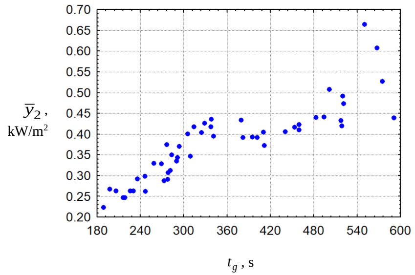
3.15 pav. Taškinės porų (t_{gl}, \bar{Q}_{FDS,l}) , (t_{gl}, \bar{y}_{1l}) ir (t_{gl}, \bar{y}_{2l}) ( l = 1, 2, \dots, 50 ) diagramos
