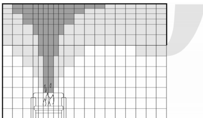
1.2 pav. Modeliuoto gaisro patalpoje modelio suskaidymas į daugybę „skaičiuojamųjų kubelių“ (Karlsson & Quintiere, 2000)
