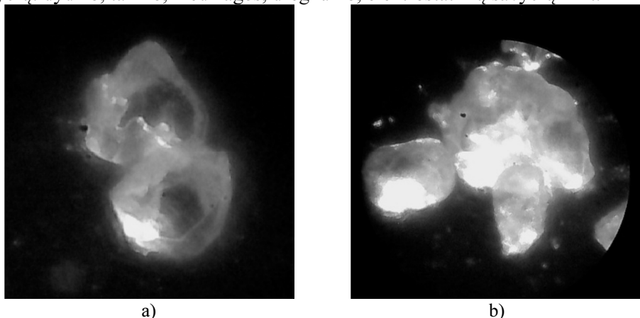
3.7 pav. Kvarcinio smėlio dalelių agregacija po akustinio lauko poveikio (vaizdas padidintas 600 kartų): a) dviejų dalelių agregacija, b) trijų dalelių agregacija
