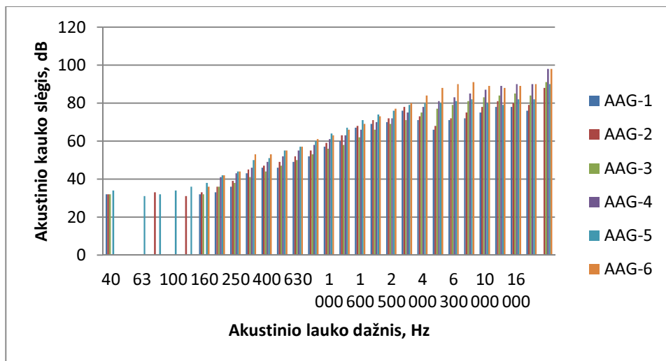
2.13 pav. Aerodinaminių akustinių generatorių spinduliuojamas akustinis laukas skirtingais dažniais
