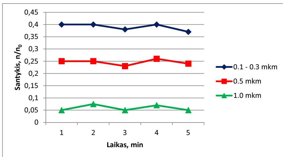
3.4 pav. Skirtingų dydžių dalelių koncentracijos pokytis oro sraute: n_0 – dalelių kiekis 1 \text{ m}^3 prieš akustinio lauko poveikį, n – dalelių kiekis 1 \text{ m}^3 po akustinio lauko poveikio
