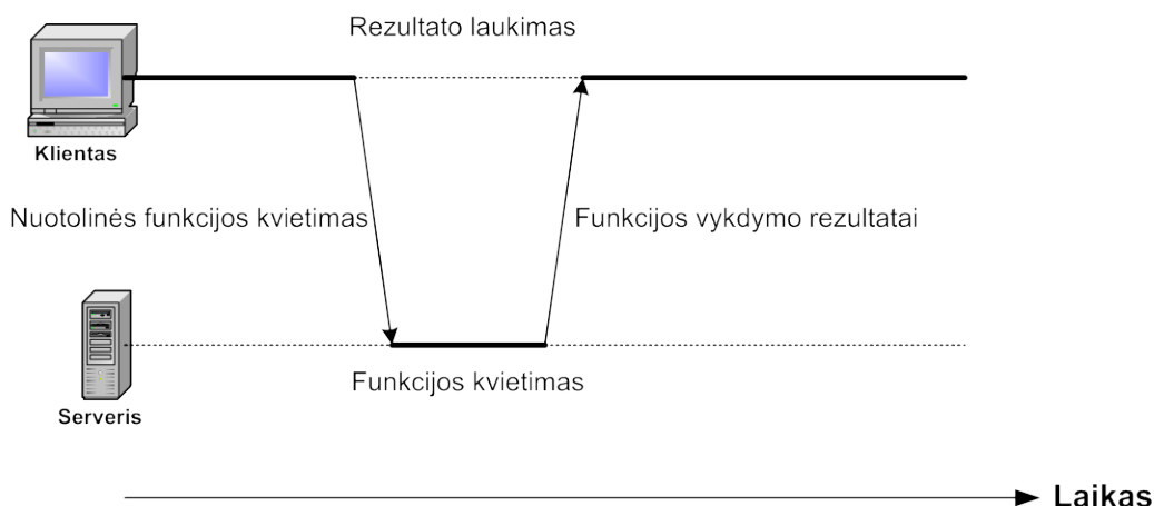
1 pav. Tipinis nuotolinės funkcijos kvietimas ir vykdymas.
