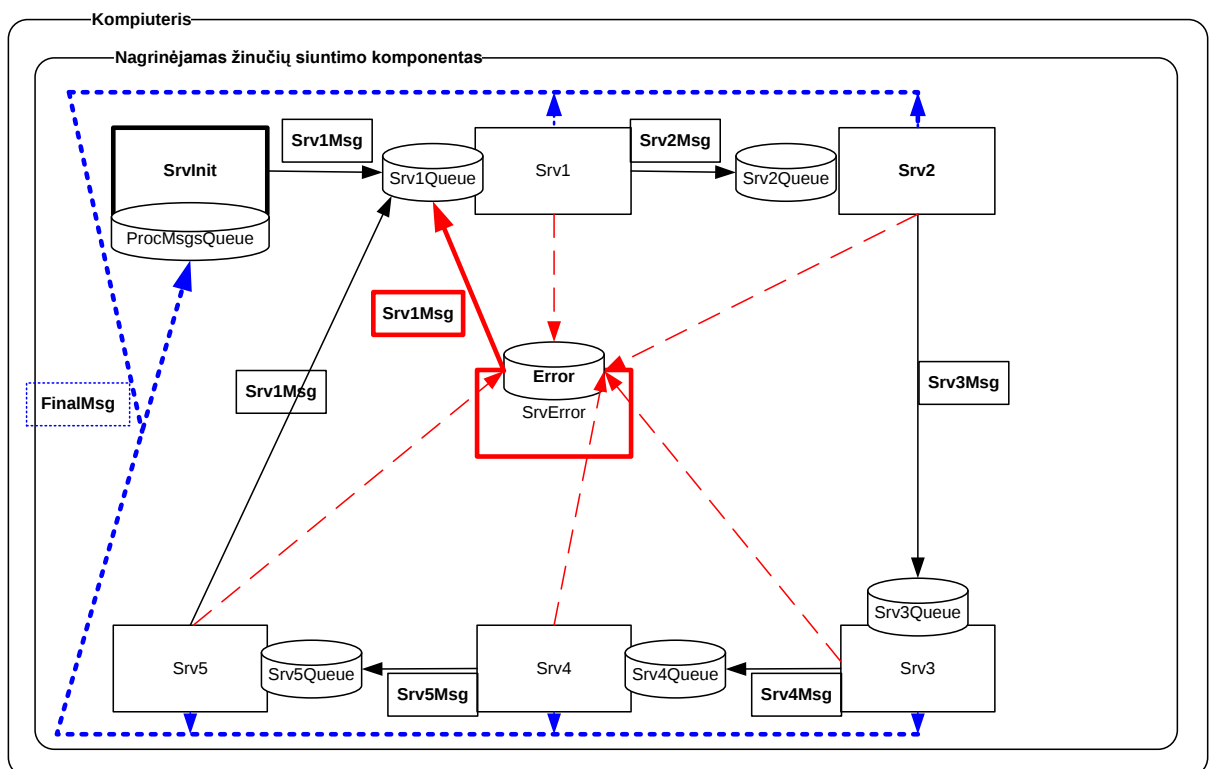
15 pav. Žinučių siuntimo ir servisų išdėstymo schema, kada nagrinėjamas užklausos/atsako siuntimas.
