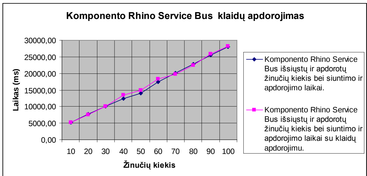
21 pav. Rhino Service Bus veikimas imituojant klaidas ir palyginimas su normaliu veikimu.
