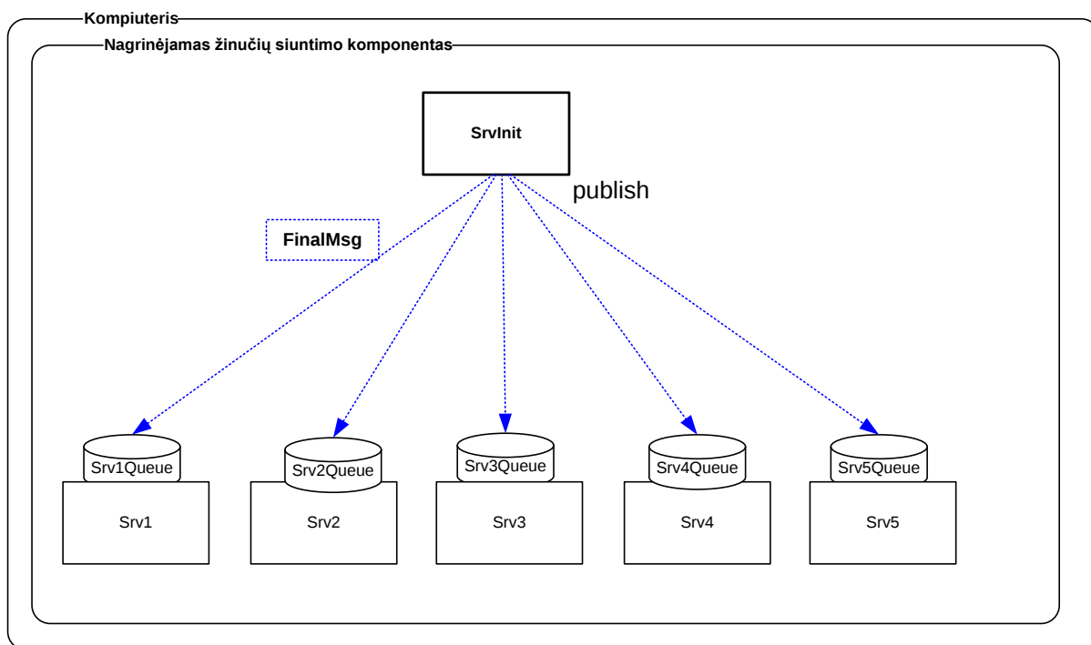
17 pav. Žinučių siuntimo ir servisų išdėstymo schema, kada nagrinėjamas transliavimo-prenumeravimo siuntimas.
