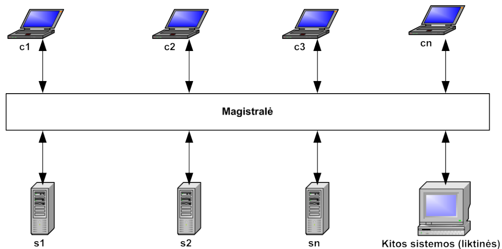
2 pav. Įmonės servisų magistralė.
