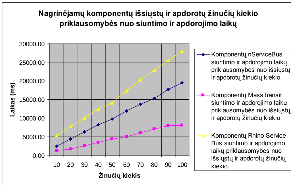
22 pav. Komponentų nServiceBus, MassTransit, Rhino Service Bus vykdyto siuntimo užklausos/atsako metodu palyginimas.
