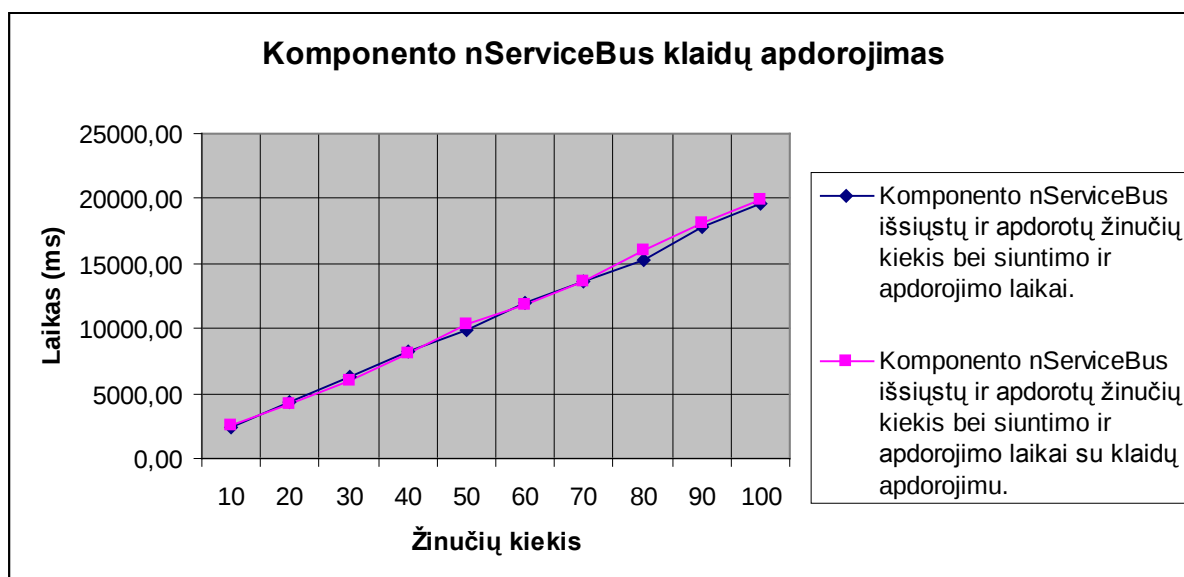
19 pav. nServiceBus veikimas imituojant klaidas ir palyginimas su normaliu veikimu.
