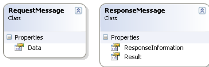
11 pav. Paketas „Messages“ skirtas duomenis ir rezultatams.
