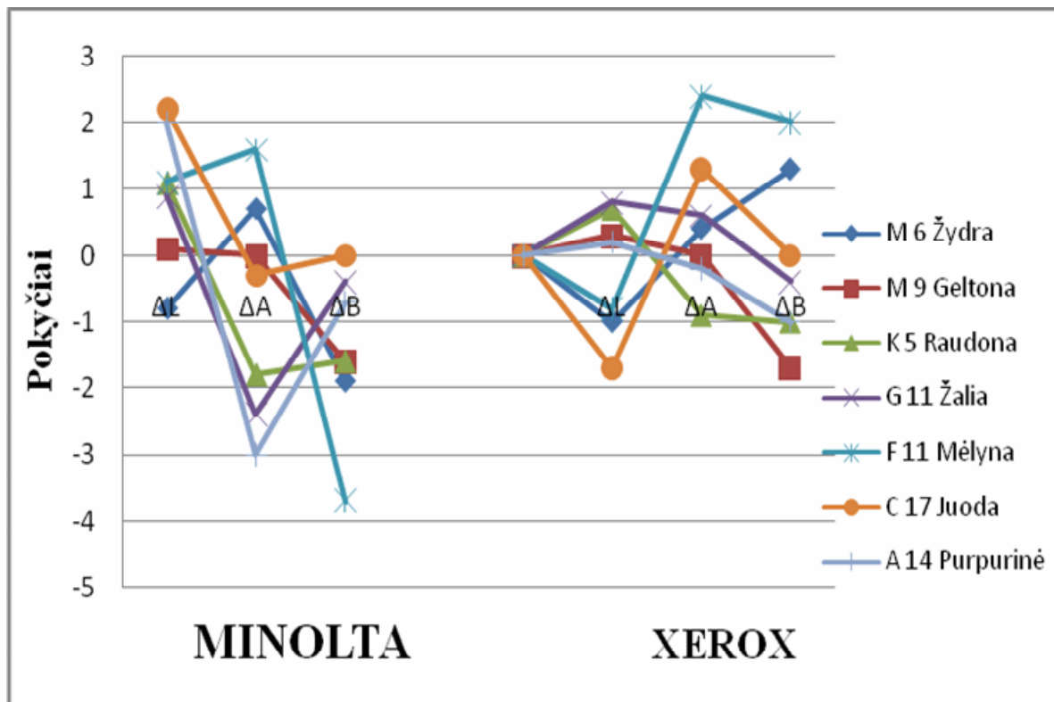
3.6 pav. Spaudos mašinų „Minolta Bizhub C6500“ grafikas iš kairės ir „Xerox DC5000“ grafikas iš dešinės, gautų spaudinių parametru \Delta L , \Delta a ir \Delta b pokyčių tarp antros ir trečios tyrimo dienos grafikas
