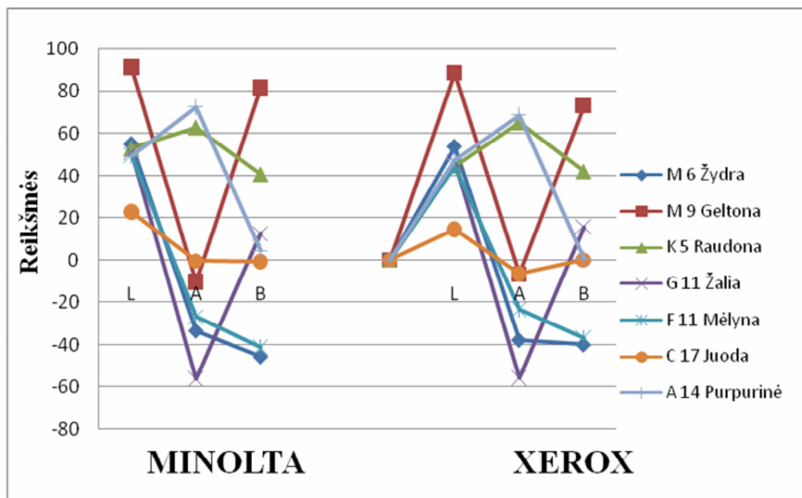
10 pav. Spaudos mašinų „Minolta“ ir „Xerox“ gautų spaudinių parametų Lab penktosios tyrimo dienos (darbo pabaigoje) grafikas
