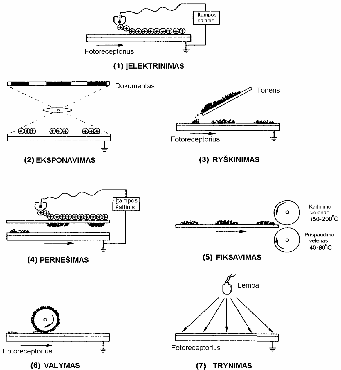
1.2 pav. Elektrofotografinio proceso etapai:
