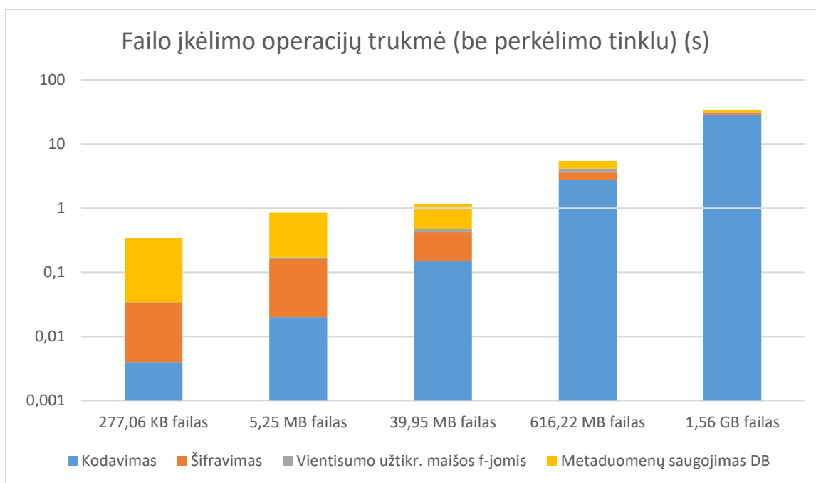
4.7 pav. Failo įkėlimo skirtingų operacijų trukmė, neskaičiuojant perkėlimo tinklu (s)
