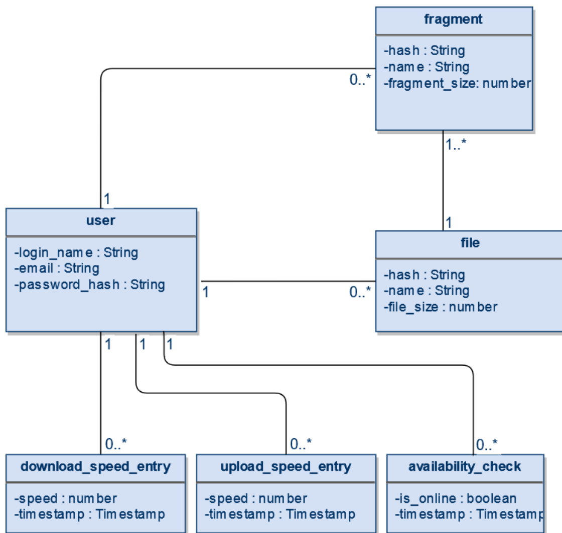
2.4 pav. Projektuojama duomenų bazės struktūra
