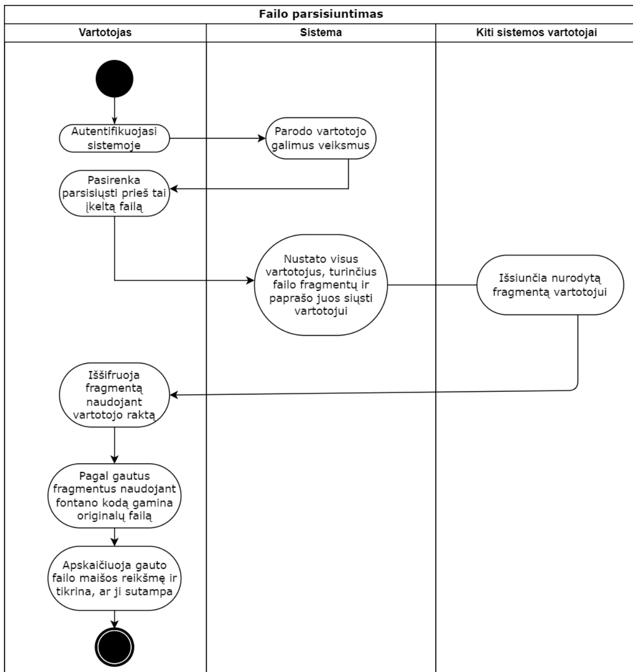
2.6 pav. Failo parsisiuntimo scenarijaus veiklos diagrama
