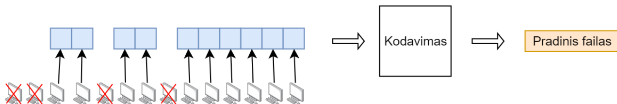
3.4 pav. Failo gavimo iš parskirstytos saugyklos schema
