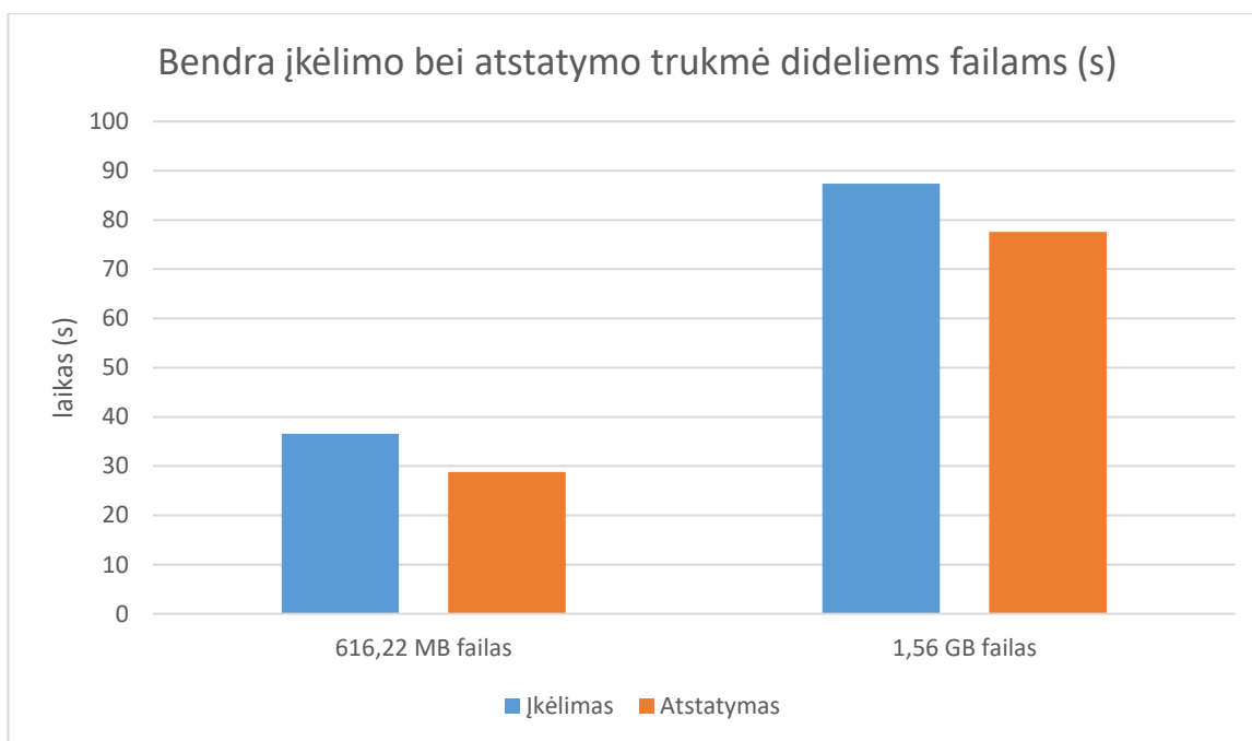
4.10 pav. Didelio dydžio failų bendras įkėlimo bei atstatymo laikas (s)
