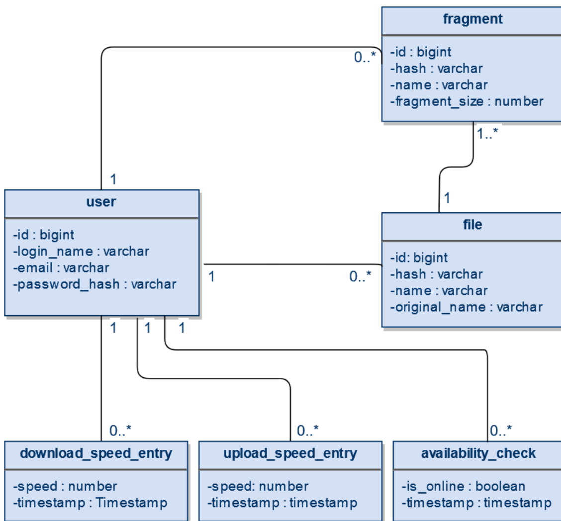
3.5 pav. Efektyvaus saugojimo paskirstytoje saugykloje metaduomenų duomenų bazės struktūra
