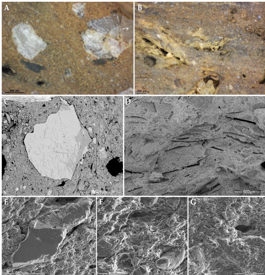
70 pav. Vėlyvai plonasienei keramikai būdinga tankinta molio masė su gausiais smulkaus kvarco grūdeliais, matoma stereomikroskopinėse (A, B), SEM-EDS BSE (C) ir SEM-EDS SE (D–G) nuotraukose. A – CW-L_M4 , kvarco (skaidrūs), feldšpatų (balti, rožiniai), raginukės (juodi) ar žėručio fragmentai ir apvalios ertmės, likusios galbūt nuo šerių ar varpos akuotų; B, D – HG-L_B1 , augalų fragmentų paliktos ertmės; C – CW-L_M4 , molio masėje matomi smulkūs kvarco ir feldšpatų grūdeliai, centre – šarminis feldšpatas (pertitas), viršuje – raginukės fragmentas, dešinėje – organikos palikta apvali juoda ertmė; E – CW-L_M4 , šarminis feldšpatas (pertitas) ir porėta molio masė; F – CW-L_M4 , porėta molio masė su apaugusiais mineralais ir, palyginimui, G – tokia pat masė šukės CW-E_M3 viršutiniame išoriniame sluoksnyje.
