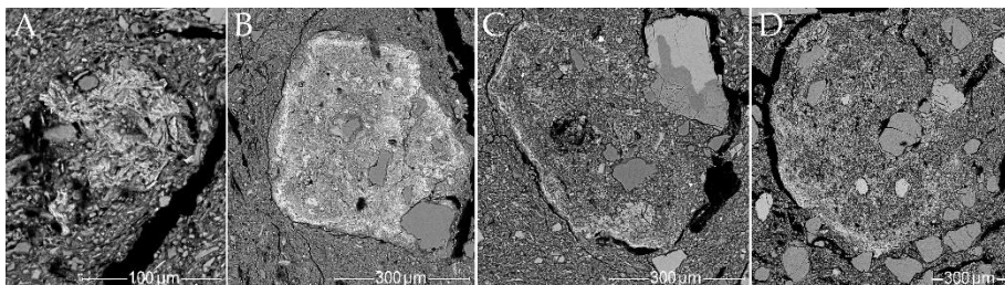
60 pav. Geležingų molio kongrecijų SEM-EDS BSE nuotraukos: A – 1000x didinimo nuotraukoje matoma žėrutinė struktūra (CW-E_M1); B – labai žemoje temperatūroje išdegta molio masė (CW-E_M3); C – žemoje temperatūroje išdegta molio masė (HG-E_M5); D – vidutinėje temperatūroje išdegta molio masė (CW-E_M1).
