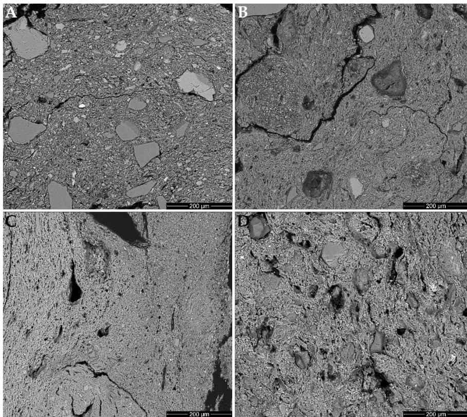
59 pav. Molio masės tekstūra SEM-EDS BSE nuotraukose. Klastinis molis su matomais adatos formos žėručiais ir įvairiais aleurito frakcijos felziniais bei akcesoriniais mineralais: A – šukė HG-E_M5 ; B – virvelinės keramikos mėginys CW-E_M2 , viršutiniame kairiajame kampe matomas kitokio molio gumulėlis (šamotas?), kurio viršutinė dalis yra identiškos struktūros kaip pagrindinė masė, o apatinė dalis su gausiais kvarco ir feldšpatu mineralais; C – brandus nuosėdinis molis su būdinga kempinė primenančia tekstūra mėginyje HG-L_B3 ; D – nuosėdinis molis su turbūt natūraliai jame susiklosčiusiais apzulintais kvarco ir feldšpatų mineralais mėginyje CW-L_M4 .
