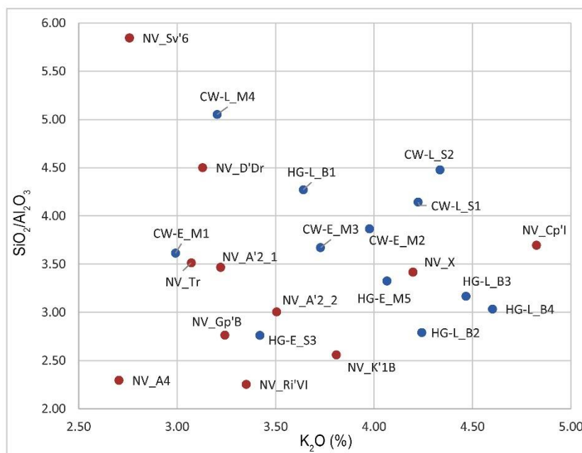
48 pav. Mėginių pasiskirstymas pagal silicio ir aliuminio oksidų santykį ir kalio oksido procentinį kiekį. Mėlyni taškai – Pietryčių Lietuvos šukės, raudoni – Narvos kultūrai priskirtinos šukės iš Rytų Baltijos regiono gyvenviečių: NV_Sv'6 – Šventosios 6; NV_Tr – Turlojiškių; NV_A2 – Asaveco 2 (Baltarusija); NV_A4 – Asaveco 4 (Baltarusija); NV_Ri'VI – Riigikula VI (Estija); NV_Cp'I – Kopu I (Estija); NV_Gp'B – Gipka B (Estija); NV_D'Dr – Dubičių-Draciliškės 1; NV_K'1B – Kretuono 1B; NV_X – eksperimentinė replika.
