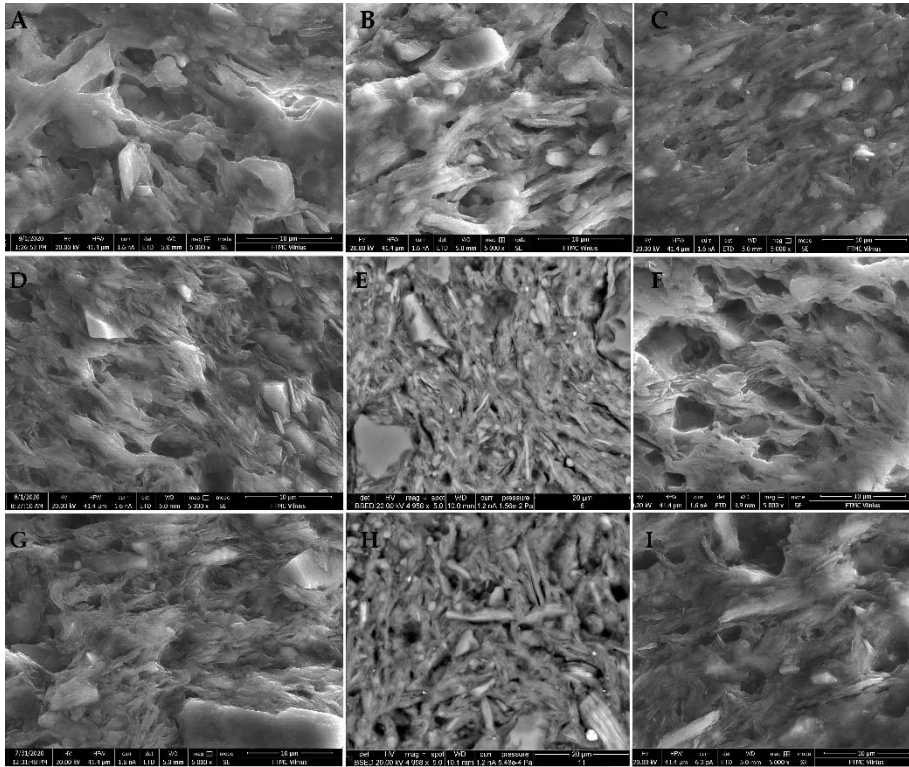
58 pav. Keramikos tekstūra SEM-EDS SE (A–D, F, G, I) ir BSE (E, H) 5000x nuotraukose. Pradinė vitrifikacija (PV): A – CW-E_M1. Stadija iki pradinės vitrifikacijos (+NV): B – HG-E_M5; C – HG-E_S3. Nevitrifikuota (NV): D – HG-L_B3; E – CW-L_S2; F – HG-L_B4; G – CW-E_M3; H – CW-E_M2; I – HG-L_B2.
