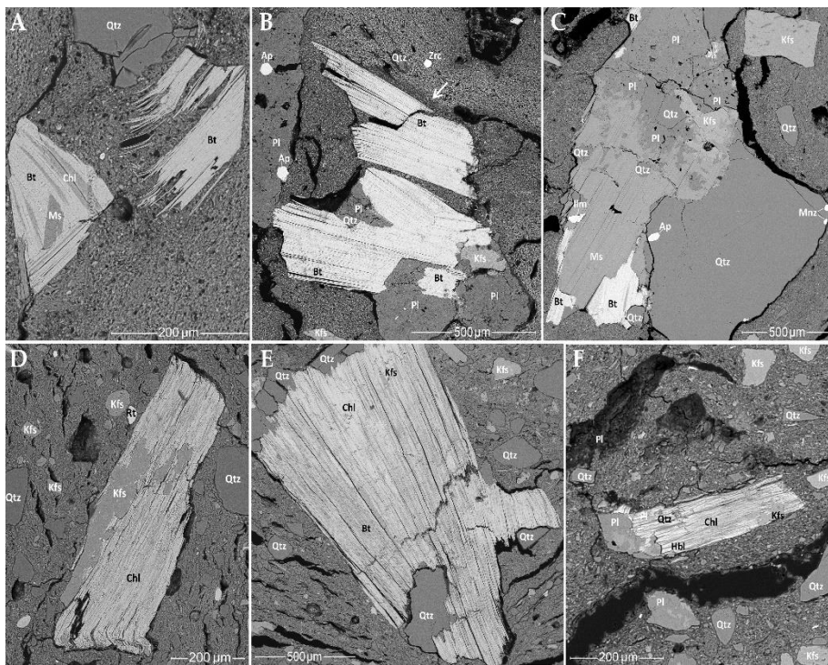
65 pav. Žėručių SEM-EDS BSE nuotraukos šukėse: A – HG-L_B3 , biotito aliteracija į muskovitą ir chloritą; B – HG-L_B3 , rodyklė žymi dėl geležies nutekėjimo iš biotito pasikeitusią molio tekstūrą; C – HG-L_B4 , biotito ir muskovito mineralai stambiame uolienos fragmente; D – CW-L_S1 , termiškai paveiktas stambus chloritas; E – CW-L_S1 , didžiausias keramikoje aptiktas žėrutis – chloritas su vietomis dar išlikusiu biotitu; F – HG-E_S3 , sudūlėjęs raginukės, aliteravusios į chloritą, fragmentas. Santrumpos: Ap – apatitas, Bt – biotitas, Chl – chloritas (šamozitas), Hbl – raginukė, Ilm – ilmenitas, Kfs – kalio feldšpatas, Mnz – monacitas, Ms – muskovitas, Pl – plagioklasas, Qtz – kvarcas, Zrc – cirkonas.
