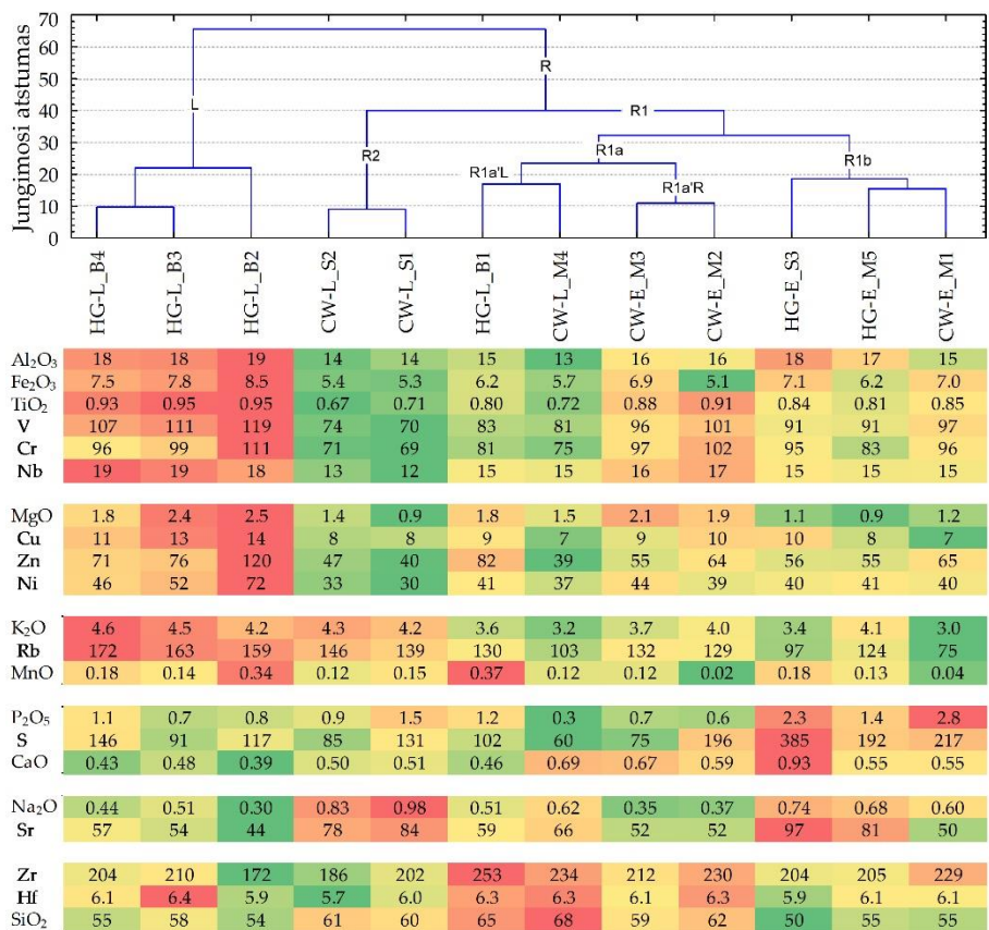
53 pav. Pietryčių Lietuvos mėginių grupavimui pagal 10 pagrindinių elementų ir 11 mikroelementų parengta klasterių dendrograma taikant Wardo metodą su miesto kvartalo atstumu. Elementų kiekiai sąlyginai suformuotoje spalvų skalėje pateikiami pagal elementų tarpusavio grupavimosi seką (pagrindinių elementų kiekiai išreikšti oksidais (%), mikroelementai – \mu\text{g g}^{-1} (aut. R. Taraškevičius).
