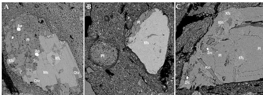
64 pav. Dūlėjimo procesų paveiktų plagioklazų SEM-EDS BSE nuotraukos: A – HG-L_B4 , granito fragmente matomas mineralams būdingas skirtingas dūlėjimo laipsnis – kvarcas (Qtz), muskovitas (Ms), kalio feldšpatas (Kfs) ir apatitas (Ap) turi aiškius konkūrus, o plagioklazo (Pl) tekstūra pakitusi, tačiau centre dar išlikusi taisyklinga oligoklazo stehiometrija; B – CW-E_M3 , apvalus albitas (Pl) grūdelis virsta moliu; C – CW-E_M1 , padūlėjęs oligoklazas (Pl) su kalio feldšpatu (Kfs) ir kaolinito (Kln) plotais.
