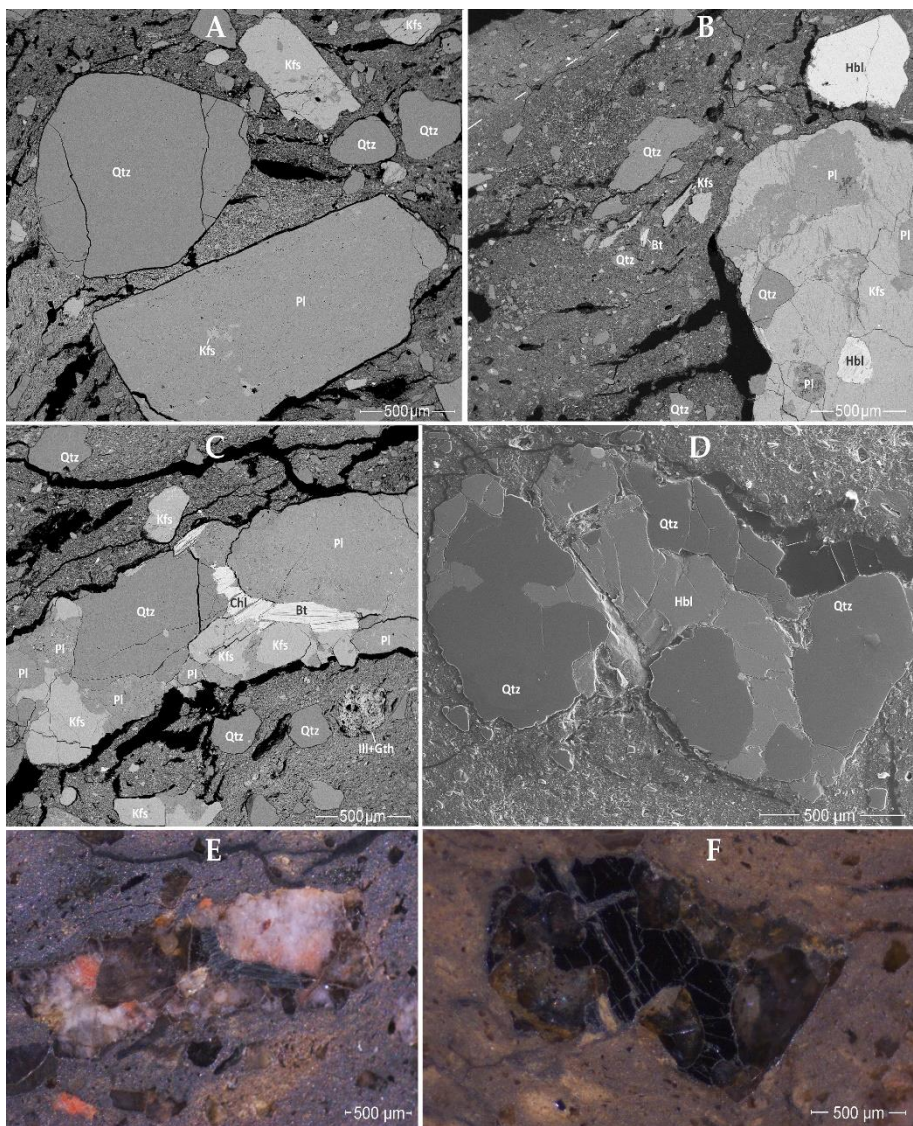
66 pav. Ankstyvosios grubios keramikos masė su mineralinėmis priemaišomis ir stambiais erdmėmis, matoma SEM-EDS BSE (A–C), SE (D) ir stereomikroskinėse (E, F) nuotraukose: A – CW-E_M1 masė su atskirais kvarco ir feldšpatų mineralais; B – HG-E_S3 masė su granito fragmentais, punktyrinė linija viršutiniame kairiajame kampe rodo ribą tarp pagrindinės masės ir viršutinio tankinto, fosforu praturtinto molio sluoksnio; C, E – HG-E_M5 masė su geležingo molio kongrecija (Ill+Gth) bei stambiu granito fragmentu, ir stereomikroskopu matomas tos pačios vietos vaizdas; D, F – HG-E_S3 granito fragmento su raginuke ir kvarcu SEM-EDS SE ir stereomikroskopo vaizdai. Santrumpos: Bt – biotitas; Chl – chloritas; Ill+Gth – getitu praturtintas ilitas; Hbl – raginukė; Kfs – kalio feldšpatas; Pl – plagioklasas; Qtz – kvarcas.
