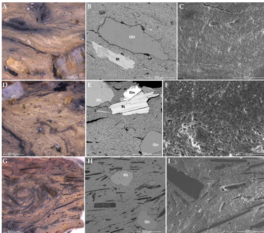
73 pav. Vėlyvosios grubios keramikos masė su plastišku smulkiagrūdžiu moliu ir stambiomis priemaišomis: A – HG-L_B3 stereomikroskopinė nuotrauka; B – HG-L_B3 , SEM-EDS BSE nuotraukoje matomas A vaizdo apatinis kairysis kampas; C – HG-L_B3 , SEM-EDS SE nuotraukoje matoma A vaizdo centrinė dalis, kurioje išsiskiria tamsesnis lygus (viršuje) ir porėtos tekstūros šviesus molis (apačioje); D – HG-L_B4 , stereomikroskopinė nuotrauka; E – HG-L_B4 , SEM-EDS BSE nuotraukoje matomas D vaizdo viršus; F – HG-L_B4 , SEM-EDS SE 1000x padidavimo nuotraukoje matomi mineraloginės sudėties skirtumai tarp tankios, tamsios, kvarco grūdėliais praturtintos ir porėtos, brandaus molio šviesios masės; G – HG-L_B2 , stereomikroskopinėje nuotraukoje matomos stambios augalų ertmės ir pavieniai smulkūs mineralai; H – HG-L_B2 , SEM-EDS BSE matoma molio masė, natūraliai patekę mineralai ir augalų paliktos ertmės; I – HG-L_B2 , augalų ertmės SEM-EDS SE nuotraukoje. Santrumpos: Bt – biotitas; Ilm – ilmenitas; Kfs – kalio feldšpatas; Qtz – kvarcas.
