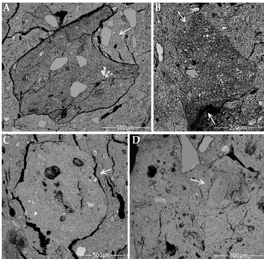
69 pav. Virvelinės keramikos masė su molio gumulėliais SEM-EDS BSE nuotraukose. Rodyklės žymi minkant molį vykstančių mechaninių deformacijų kryptis. A – CW-E_M2, tamsioje masėje šviesaus molio gumulėlis su raginukės trupiniais (balti fragmentai); B – CW-E_M2, tamsioje masėje neaiškių kontūrų šviesesnio molio gumulėlis su gausiais kvarco ir kalio feldšpato grūdeliais; C – CW-E_M3, tik kontaktinė ertmė skiria tokios pačios tekstūros molio gumulėlį nuo pagrindinės tamsios masės; D – CW-E_M3, šviesaus molio masėje pastebėti įvairiomis kryptimis orientuoti amorfiniai molio gumulėliai.
