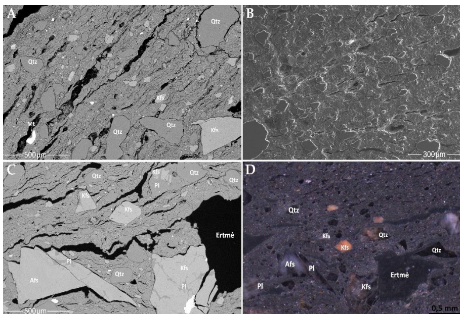
71 pav. Šakių lankos postvirvelinės keramikos juodos masės tekstūra, matoma SEM-EDS BSE (A,C), SEM-EDS SE (B) ir stereomikroskopinėse (D) nuotraukose. A, B – CW-L_S1 , juoda molio masė su gausiais tikriausiai natūraliai patekusiais smulkiais mineralais bei apvaliomis ertmėmis. C, D – CW-L_S2 , ta pati šukės vieta su matomais kampuotais granito fragmentais ir stambia neaiškios organikos (ar oro?) ertme. Santrumpos: Afs – šarminis feldšpatas (pertitas), Kfs – kalio feldšpatas, Mt – magnetitas, Pl – plagioklazas (albitas), Qtz – kvarcas.
