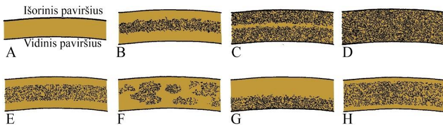
105 pav. Stilizuotos šukių pjūvių schemos, parodančios, kaip nuo išdegimo sąlygų ir organikos priklauso šviesios (gelsvo, raudono, rudo) ir tamsios (pilko, juodo) molio masės pasiskirstymas šukėje: A – oksiduota, organika pradžioje galėjo būti, bet išdegė (šerdis nėra); B – oksiduota, pradžioje buvo organika (išsklaidytos šerdis ribos); C – redukuota, organikos pradžioje nebuvo (juoda ar pilka spalva gali išsiplėsti nepalikdama šviesios šerdis); D – redukuota, pradžioje buvo arba nebuvo organikos; E – redukuota, greitai atvėsinta ore (aiškios šerdis ribos); F – marmurinė struktūra, persidengiantys oksiduoti ir redukuoti plotai; G – oksiduota, vidinis paviršius redukuotas dėl deguonies trūkumo indo viduje; H – redukuota (arba dalinai oksiduota), plonas šviesus sluoksnis dėl postdepozitinių sąlygų (A–E – pagal Rye 1981, 116; F, G – pagal Eramo, Mongone 2019, Figure 3. Modifikuota iš Rye 1981, 116, Fig. 104).
