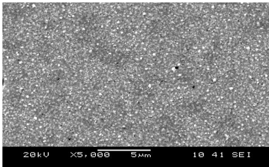
Рис. 1. СЕМ–зображення поверхні тонкої плівки Pb_{0.9}Cd_{0.1}Te:Pb зі збільшенням 5000 разів. Час наплення 80 с.
