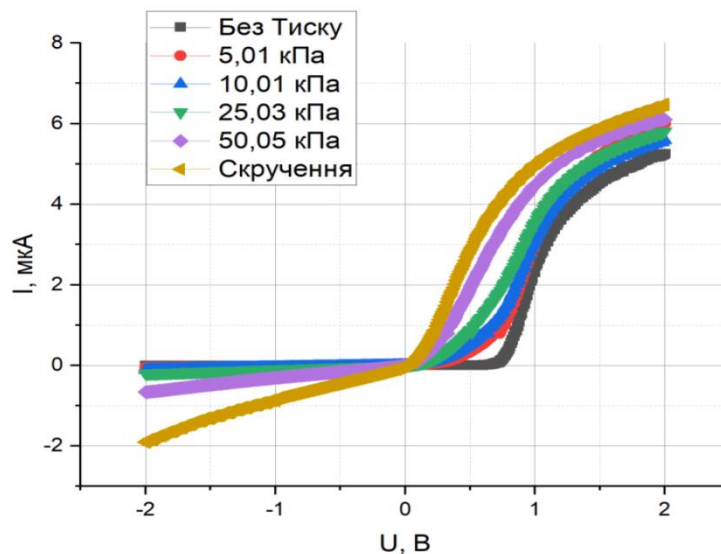
Рис.1 ВАХ структури Mo-CdS- Cu_xS без освітлення.
