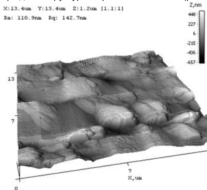
Рис.1. Морфологія поверхні кристалу CdSb після лазерної проплавки (дослідження в АСМ).
