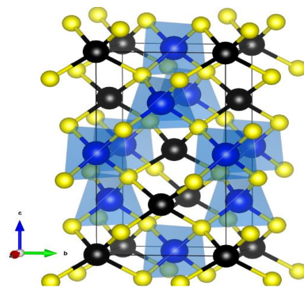
Рис. 1. Структура кристалічної ґратки для \text{AgGaS}_2 . Чорні кульки відповідають атомам Ag, жовті та сині кульки відповідають атомам S та Ga, відповідно.
