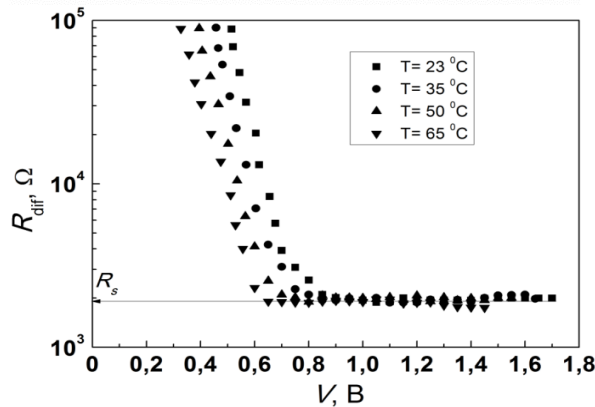
Рис. 2. Залежність диференційного опору структури графіт/p-InP від напруги при різних температурах
