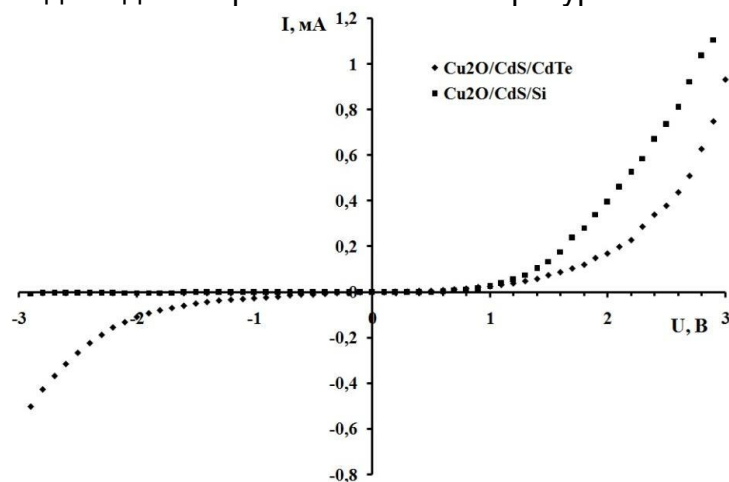
Рис. 1. ВАХ гетероструктур \text{Cu}_2\text{O}/\text{CdS}/\text{Si} та \text{Cu}_2\text{O}/\text{CdS}/\text{CdTe}
