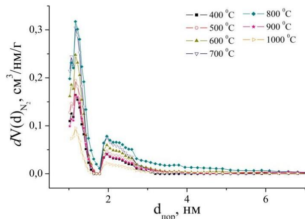
Рис. 2. Розподіл пор за розмірами за методом DFT (Density Functional Theory) [4]
