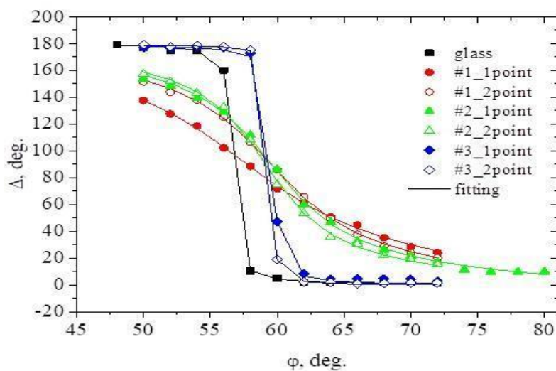
Рис. 2. Залежність еліпсометричного кута \Delta від \phi .
