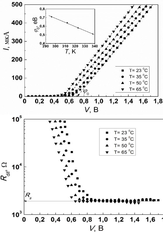
Рис. 2. Залежність диференційного опору структури графіт/p-InP від напруги при різних температурах
