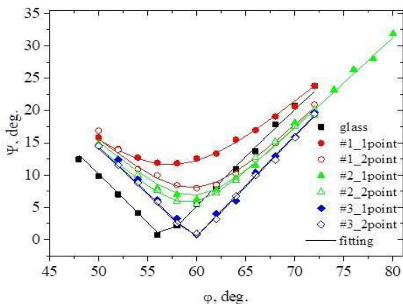
Рис. 1. Залежність еліпсометричного кута \psi від \phi .
