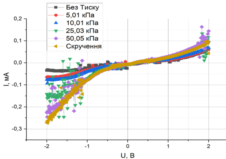
Рис. 2. ВАХ структури Mo-CdS-Cu x S при освітленні.
