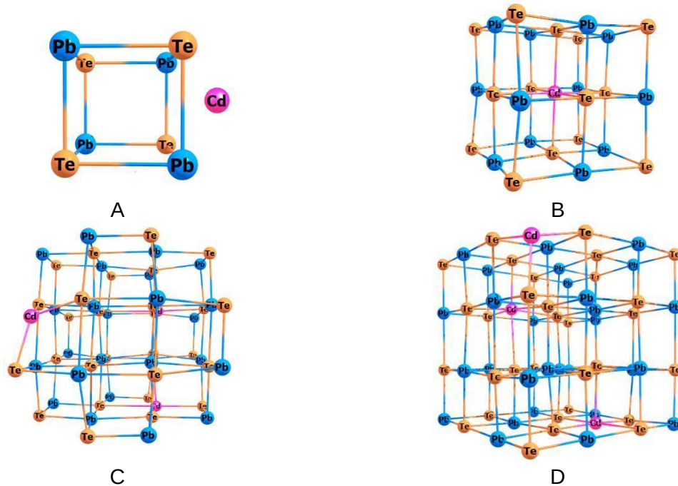
Рис. 2. Моделі кластерів PbCdTe: A) Pb_4Te_4 , B) Pb_{13}Cd_1Te_{13} , C) Pb_{25}Cd_3Te_{28} та D) Pb_{29}Cd_3Te_{32}
