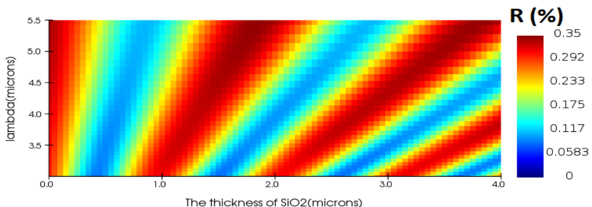
Рис.2. Графік залежності коефіцієнта відбивання від товщини силіцій оксиду в діапазоні 3-5.5мкм.
