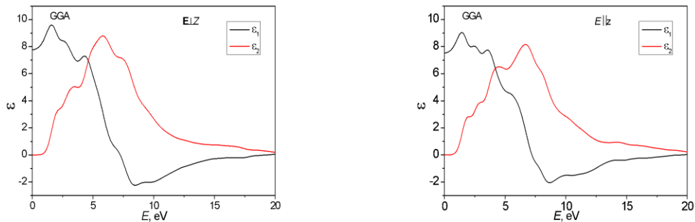
Рис. 2. Діелектрична функція кристала \text{AgGaS}_2 розрахована з використанням GGA функціоналу.
