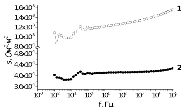
Рис. 1. Імпедансні спектри системи \text{LiMn}_{1.95}\text{Fe}_{0.05}\text{O}_4 , синтезованої при
