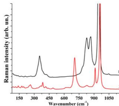
Рис.2. Спектри КРС гідрату \text{NiMoO}_4 (1) та \alpha - \text{NiMoO}_4 (2)
