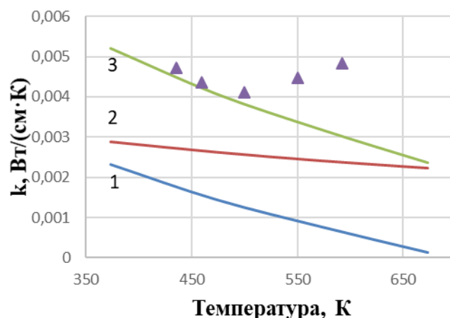
Рис. 1. Температурні залежності коефіцієнта теплопровідності k зразка Pb_{0.6}Sn_{0.4}Te (1 - k_e , електронна складова теплопровідності, 2 – k_{lat} , граткова складова, 3 - загальна теплопровідність зразка, ▲ – теплопровідність отримана експериментально [3])
