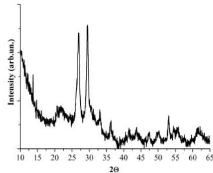
Рис.1. Х-променева дифрактограма гідротермально-отриманого молібдату нікелю
