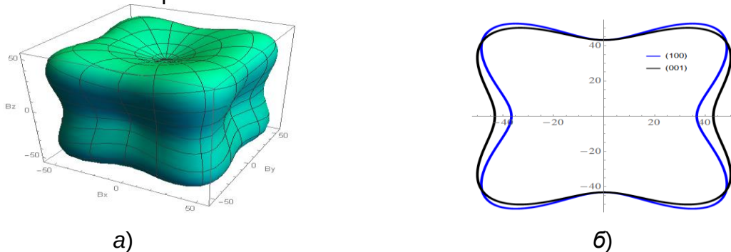
Рис. 3. 3D розподіл модуля Юнга (а), та його проекції на площини (100) та (001) (б).
