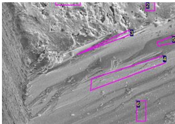
Рис.2. Морфологія після лазерної обробки поперечного перерізу епітаксійної структури на основі \text{In}_4\text{Se}_3 (дослідження в РЕМ).
