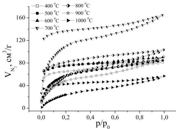
Рис. 1. Ізотерми сорбції азоту для НВМ
