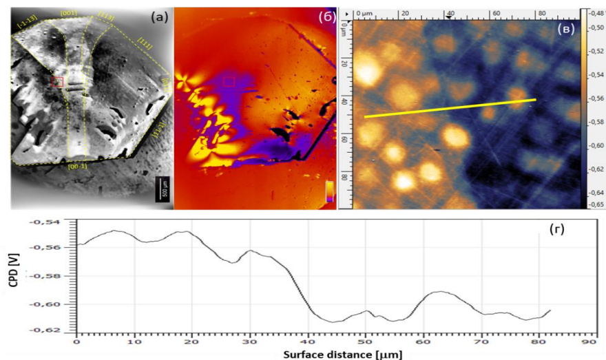
Рис.1. Оптична мікрофотографія багатосекторної підкладки напівпровідникового алмазу (а), відповідна візуалізація деформаційних полів у поляризованих променях (б). Карта поверхневого потенціалу (в) та відповідний профіль на границі секторів {111} та {113}.
