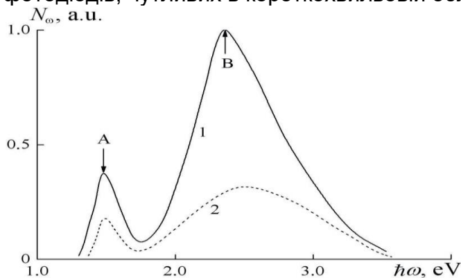
Рис. 1. Спектри фотолюмінесценції для підкладок CdTe:O із 1) вільною поверхнею та 2) покритою золотою плівкою.
