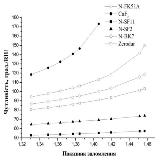
Рис.1. Залежність чутливості від показника заломлення водних розчинів гліцерину для різних матеріалів призм
