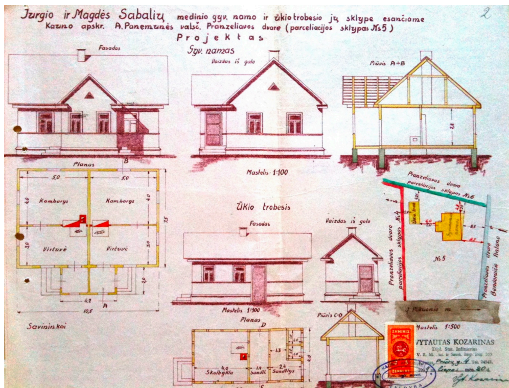
45 pav. J. ir M. Sabalių gyv. namo projektas Prendzialivos dv., A. Panemunės v. 1939 m.
