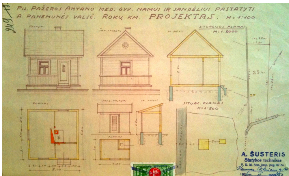
40 pav. Pažeros Antano gyv. namo projektas Rokų k., A. Panemunės v.
