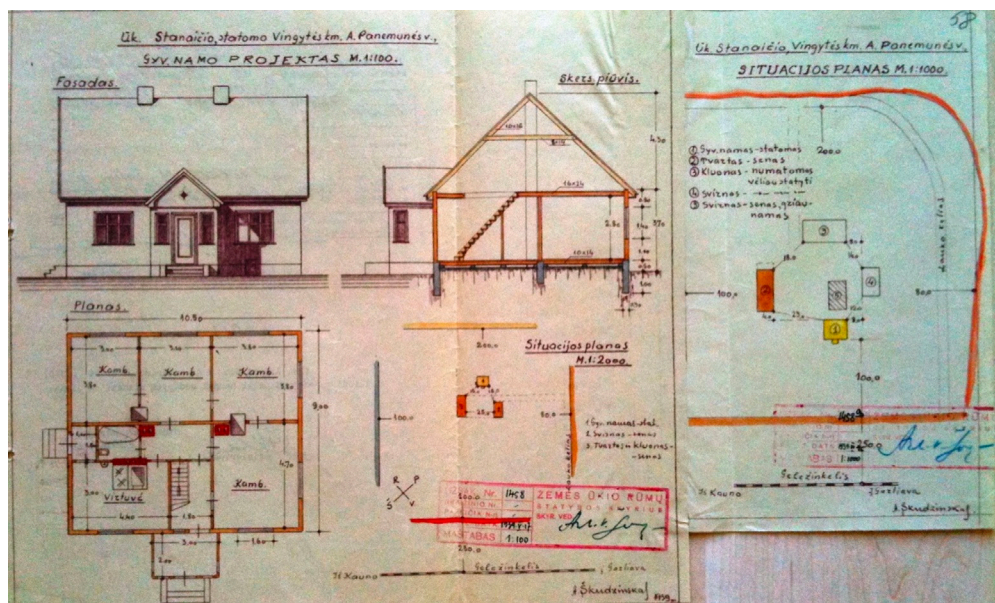
46 pav. Pil.. Stanaičio Kompaktiško plano gyv. namo projektas Vingytės k., A. Panemunės v. 1934 m. KRVA, f. 17, b. 26–58
