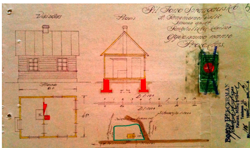
39 pav. Jono Sprangauskio gyv. namo projektas Pakalniškių k., A. Panemunės v.
