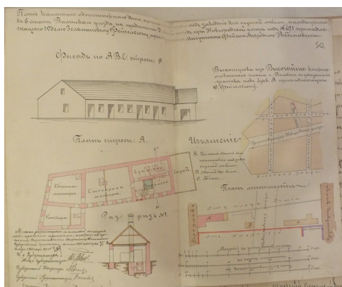
116. Feigos Rabinovič lenktųjų baldų fabriko projektas, 1900
