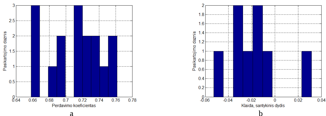
5.20 pav. Pirmojo kanalo perdavimo koeficiento (a) ir prognozavimo klaidos (b) histogramos taške 20 GHz
