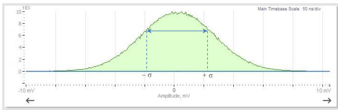
4.5 pav. Triukšmo įtampos matavimo histograma esant tuščiam strobavimo įtaiso įėjimui
