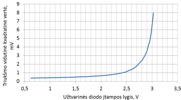
1.7 pav. Išmatuota strobavimo grandinės triukšmo jėgime priklausomybė nuo užtvarinės įtampos
