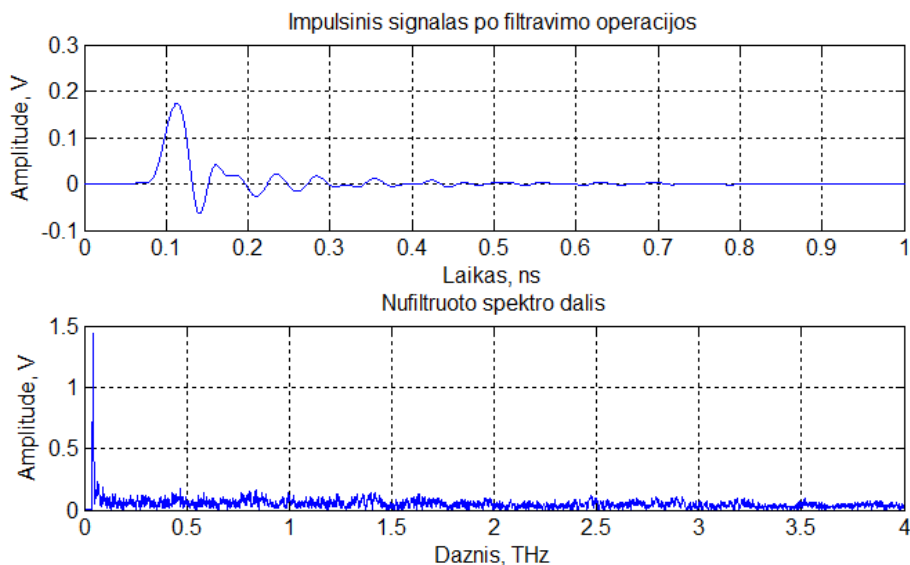
5.12 pav. Impulsinio signalo filtravimo procedūros rezultato ir nufiltruoto triukšmo spektro grafikai
