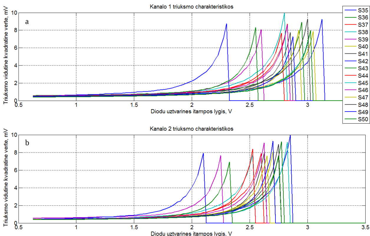
5.17 pav. Triukšmo S1 pirmo (a) ir antro (b) kanalų įėjimuose priklausomybė nuo diodų užtvarinės įtampos lygio
