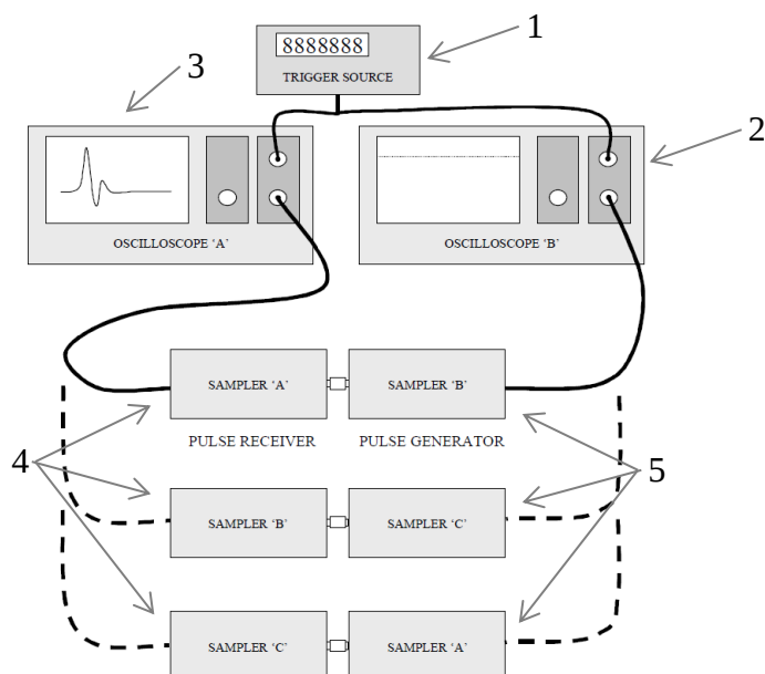
2.1 pav. Trijų storbuojančių osciloskopų sistema dažninės charakteristikos matavimui taikant priešpriešiais sujungtų strobavimo grandinių metodą. Čia 1 – synchronizacijos signalo šaltinis; 2 – osciloskopas, veikiantis kaip generatorius; 3 – osciloskopas, veikiantis kaip imtuvas; 5 ir 4 – trijų strobavimo grandžių matavimo kombinacijos, kai kiekviena yra naudojama kaip impulsinio signalo imtuvas arba generatorius. Pritaikyta iš [11]
