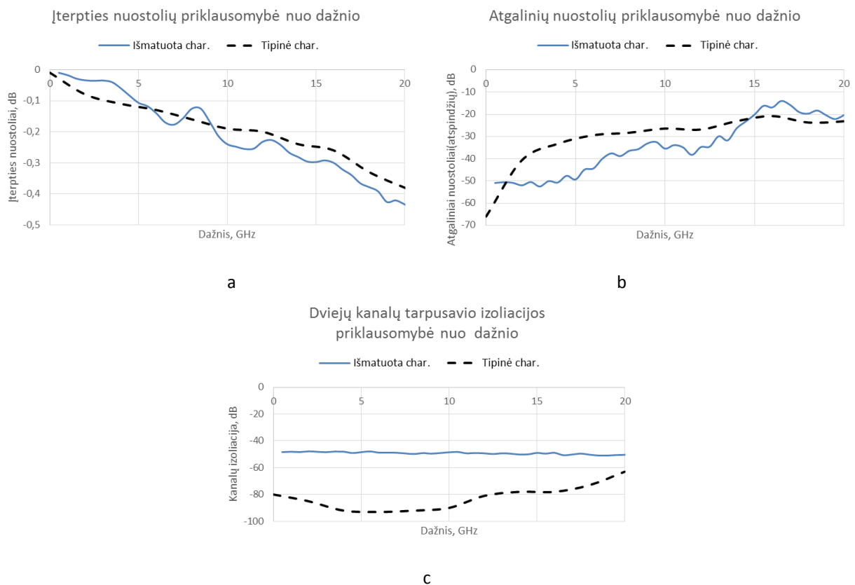
3.4 pav. Aukštadažnių relių įterpties nuostolių (a), atgalinių nuostolių dėl atspindžių nuo įėjimo (b), dviejų kanalų tarpusavio izoliacijos (c) patikros rezultatai
