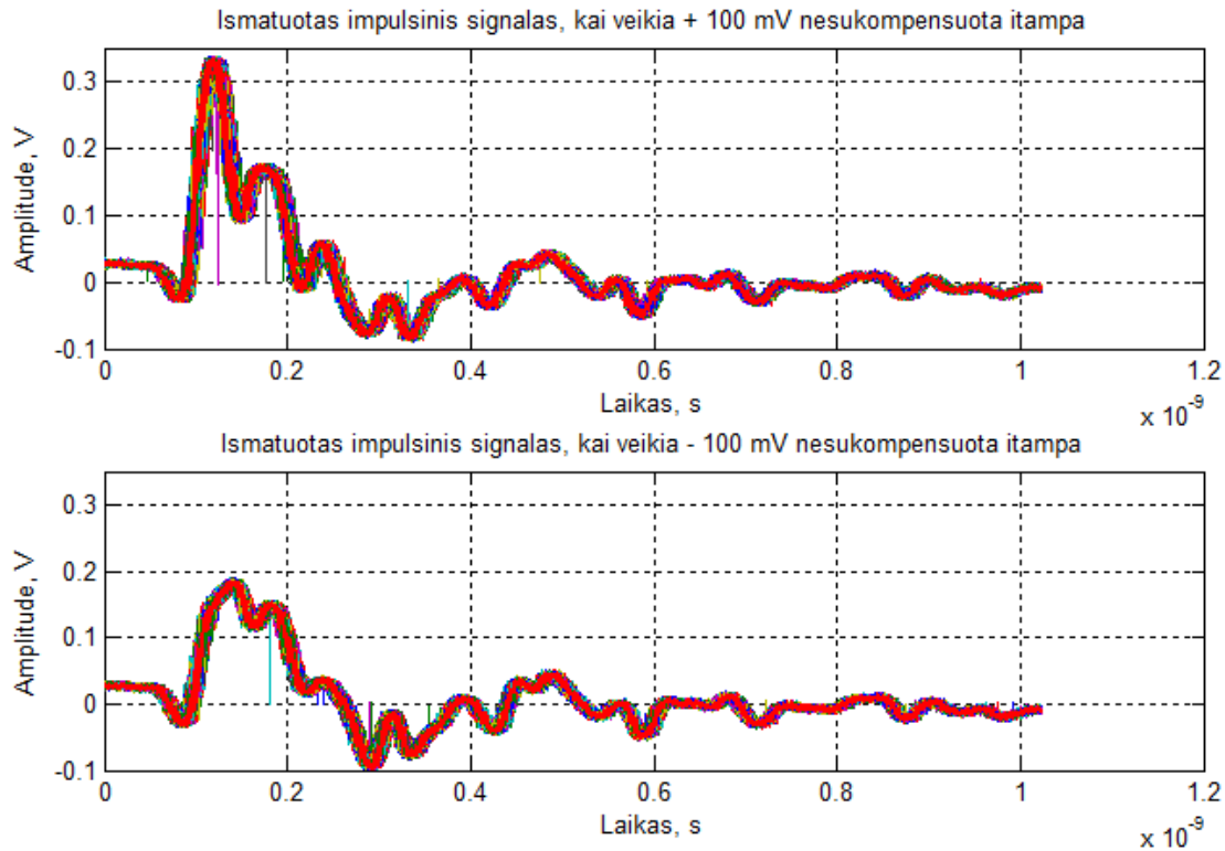
5.6 pav. Teigiamo ir neigiamo impulsinių signalų matavimo rezultatai veikiant strobavimo grandinės įėjime \pm 100 mV didžio nesukompensuotai įtampai
