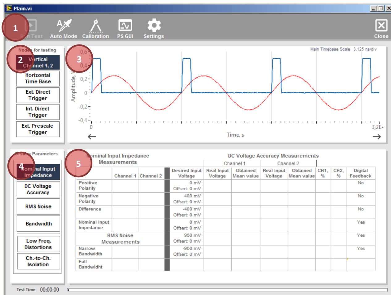
4.3 pav. ATS valdymo programos pagrindinio lango vaizdas, čia: 1 – įrankių juosta; 2 – testuojamų mazgų parinktės laukas; 3 – osciloskopu surinktų signalų imčių ir konstruojamų histogramų atvaizdavimo laukas; 4 – mazgo testuojamo parametro parinktės laukas; 5 – pasirinkto parametro matavimo rezultatų (lentelių arba/ir grafikų) atvaizdavimo laukas
