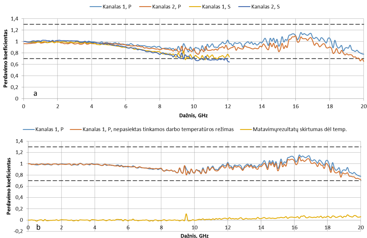
4.6 pav. Pirmojo ir antrojo kanalų DACH matavimo rezultatų grafikas, kai kiekvienas iš kanalų dirba pilnos ir siauros praleidžiamųjų dažnių juostos režimais (a), matavimų pakartojamumo patikra matuojant tą patį kanalą, kai antruoju atveju nepasiektas tinkamas temperatūrinis darbo režimas (b)
