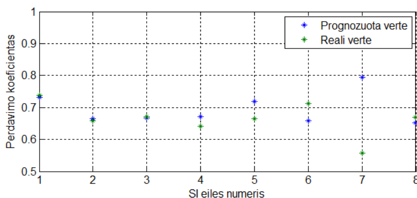
5.23 pav. Antrojo kanalo perdavimo koeficiento prognozavimo rezultatai
