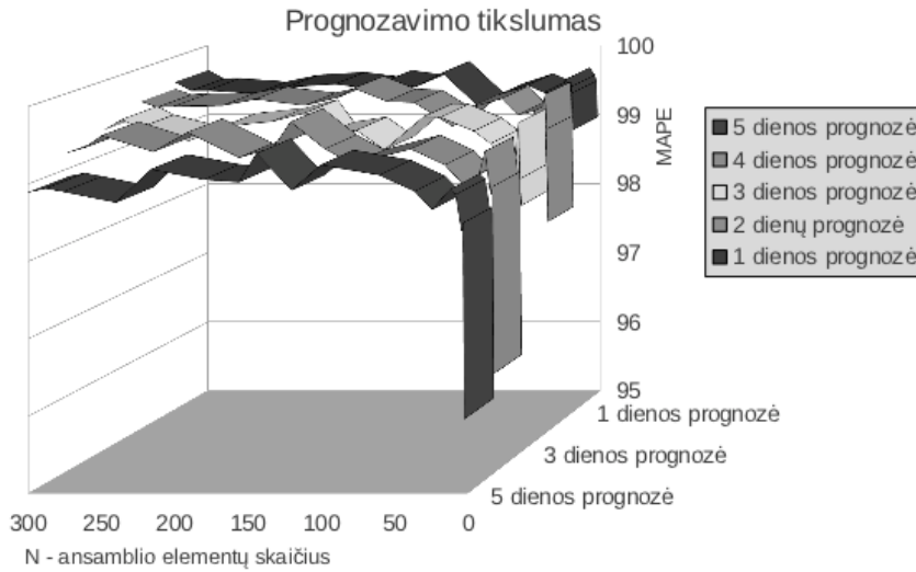
3.7 pav. Prognozavimo tikslumo priklausomybė nuo Evolino rekurentinių neuroninių tinklų skaičiaus, prognozuojant 1–5 dienas į ateitį
