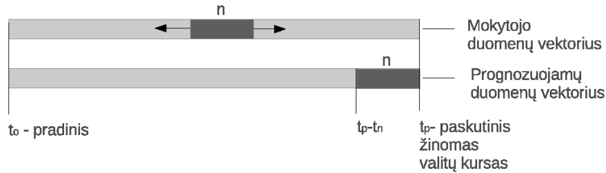
3.2 pav. Ortogonalinių įvesčių parinkimas iš prognozuojamo ir „mokytojo“ duomenų vektorių
