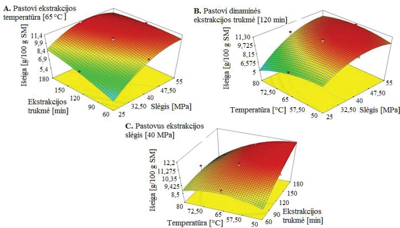
3 pav. Spanguolių išspaudų SKE-CO 2 atsako paviršiaus kreivės, parodančios ekstrakto išeigos priklausomybę nuo optimizuojamų parametru: A – nuo ekstrakcijos trukmės ir slėgio; B – nuo temperatūros ir slėgio; C – nuo ekstrakcijos trukmės ir temperatūros
