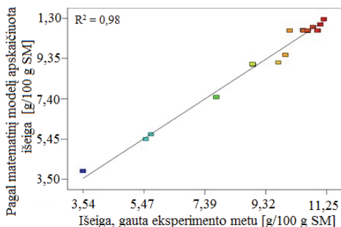
2 pav. Ekstrakto išeigos, gautos eksperimento metu ir apskaičiuotos taikant sudarytą matematinį modelį
