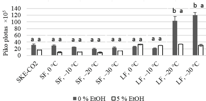
6 pav. \beta -sistosterolio kiekio pokyčiai frakcionuojant spanguolių išspaudas taikant SKE-CO 2 su tirpikliu arba be jo (5 % EtOH). SF – sunkesnioji frakcija; LF – lengvesnioji frakcija. a, b raidės tarp tos pačios spalvos stulpelių nurodo reikšmingus skirtumus (ANOVA, p < 0,05 ). Pateiktos vidutinės dviejų matavimų vertės \pm SN
