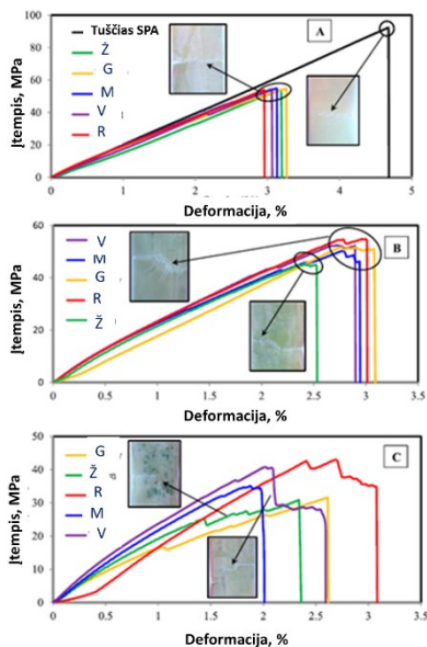
11 pav. Iš SPA ekstrahuotų stiklo pluošto bandinių įtempių ir deformacijų kreivės: A) tuščios, B) vienosės, ir C) daugiapusės SPA (spalvų kodai 1 lent. G – geltonas, Ž – žalias, M – mėlynas, R – raudonas, V – violetinis )
