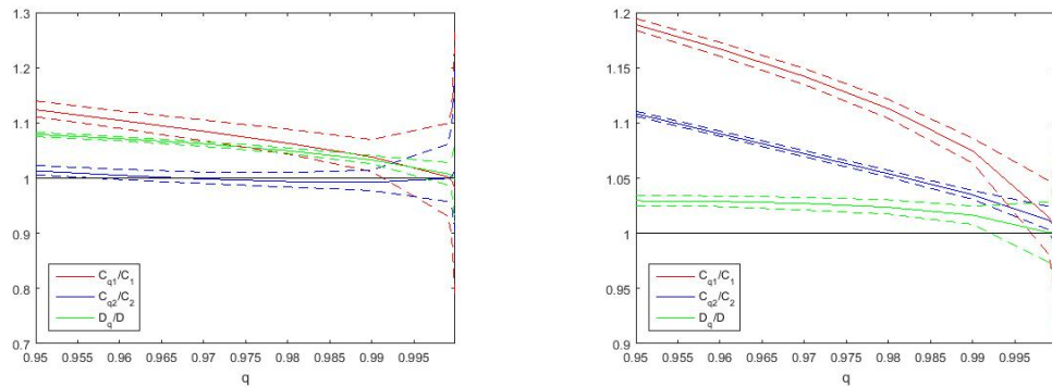
a: \nu = 2.
