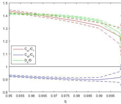
a: \rho = 0.7 .
