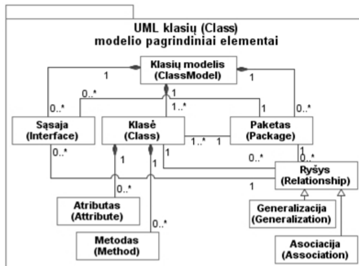
Pav. 14. Pagrindiniai UML klasių modelio elementai
