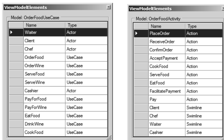
Pav. 42. Nuskaityto UML modelio elementų sąrašas
