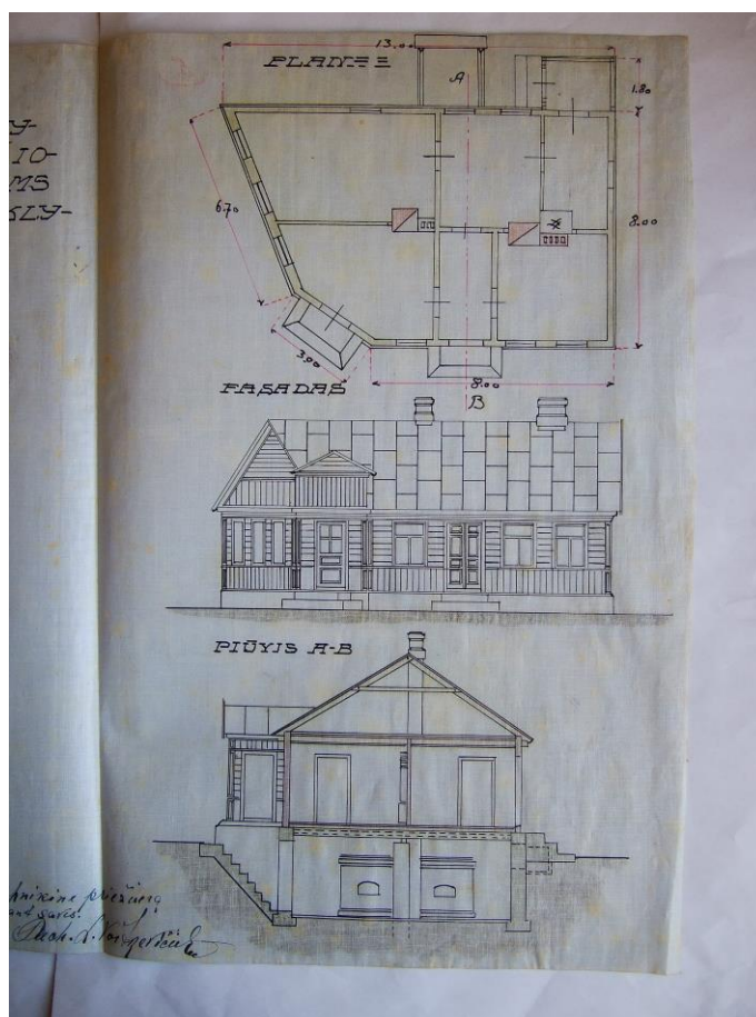
43 pav. Vokiečių g. 65; 1924 m. namo statybos projektas
