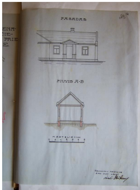
58 pav. Kranto 2 – oji g. 6; 1920 m. statyto priestato projektas
