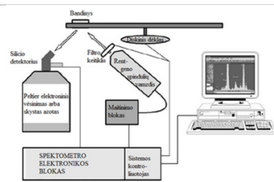
3XRF. Principinė rentgeno fluorescencinio aktyvavimo/švitinimo schema
