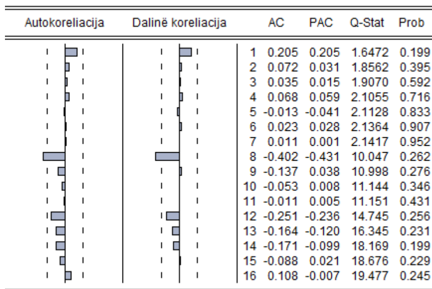
52 pav. Fiksuoto telefono ryšio linijų paklausos įvertinimo korelograma
