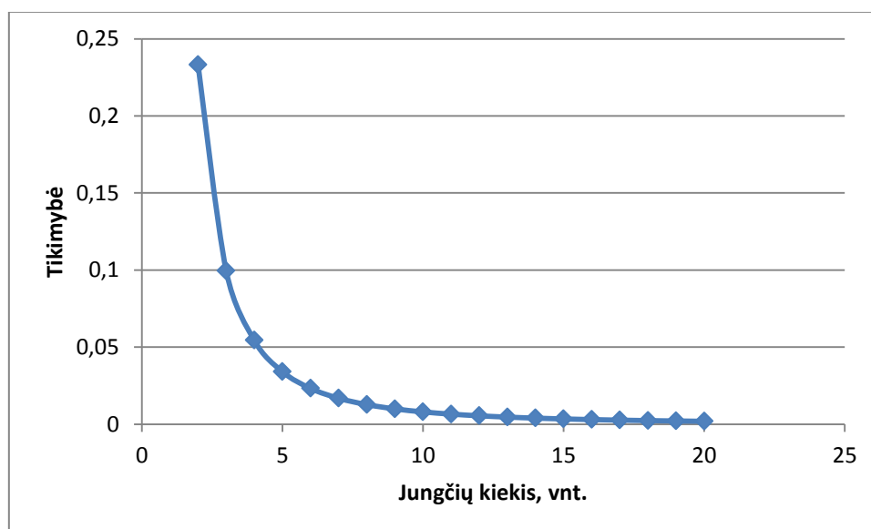
8 pav. Nuo mastelio nepriklausomo tinklo jungčių pasiskirstymas
