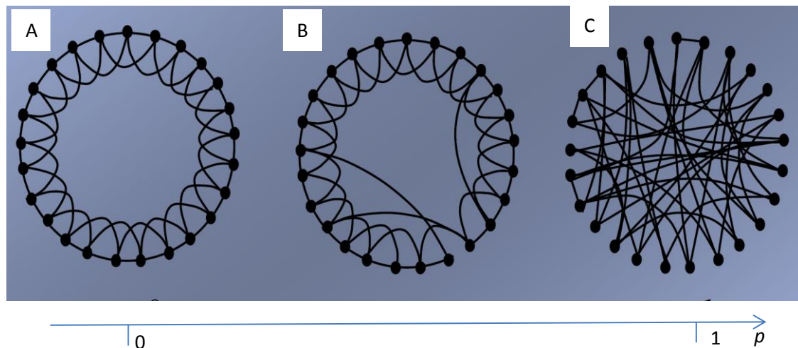
9 pav. Tinklų skirstymas pagal jungčių chaotiškumą (Watts & Strogatz, 1998)
