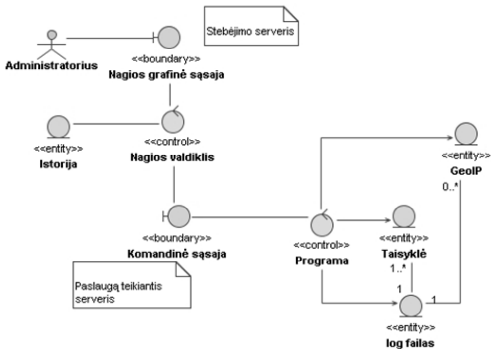
45 pav. Analizės klasių modelis
