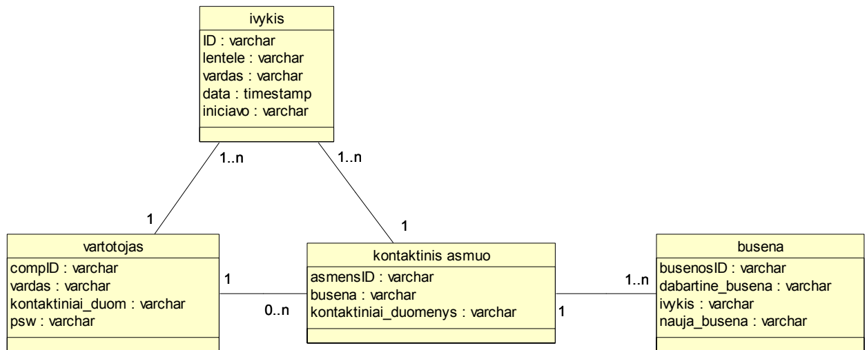
2.10 pav. Objekto „kontaktinis asmuo“ klasių diagrama
