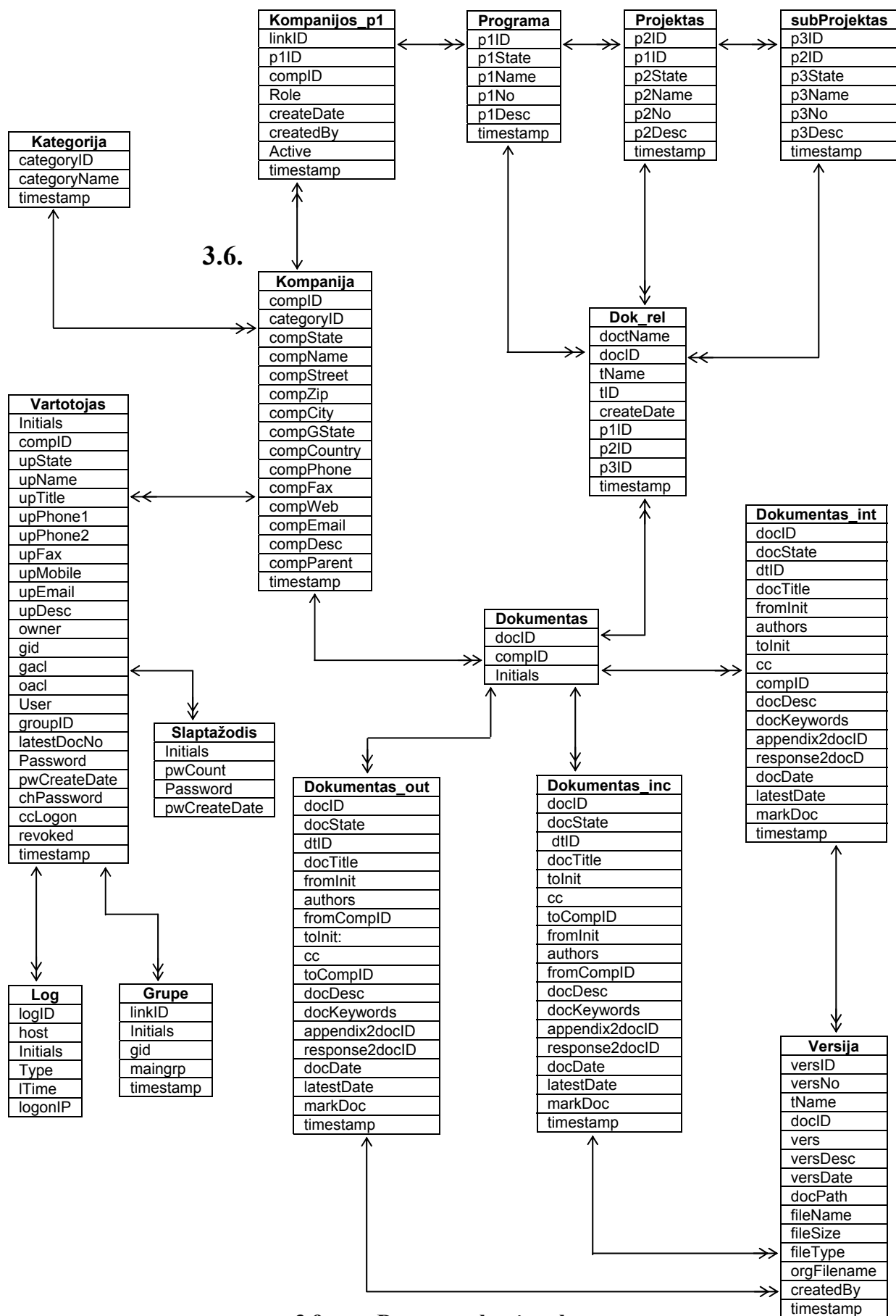
3.9 pav. Duomenų bazės schema
