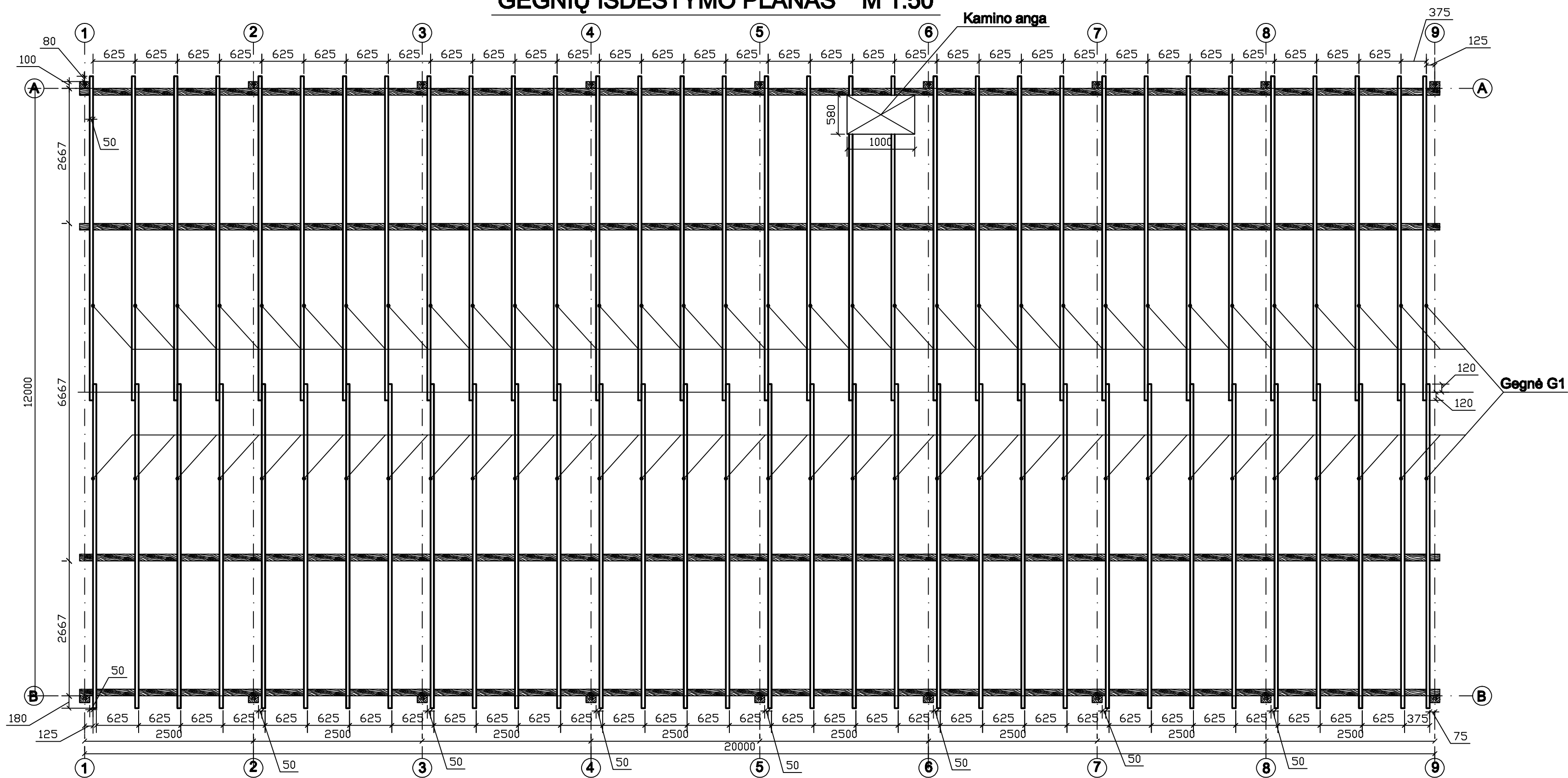
GEGNIŲ IŠDĖSTYMO PLANAS M 1:50
