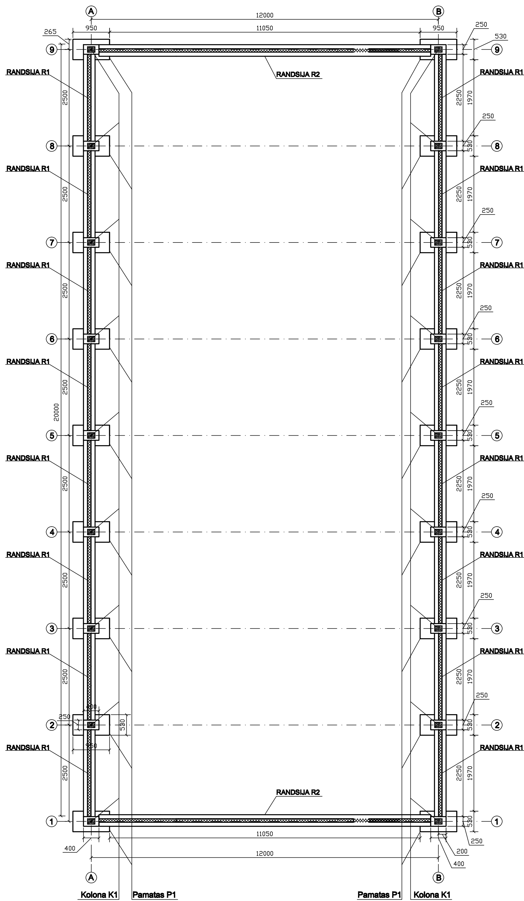
PAMATŲ IR KOLONŲ IŠDĖSTYMO PLANAS M 1:50
