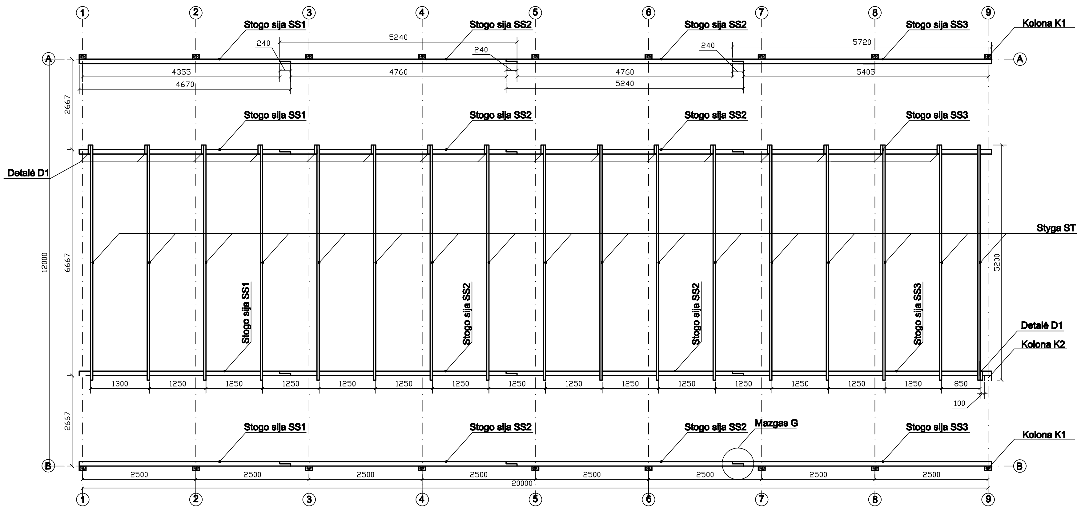
GEGNIŲ IŠDĖSTYMO PLANAS M 1:50
