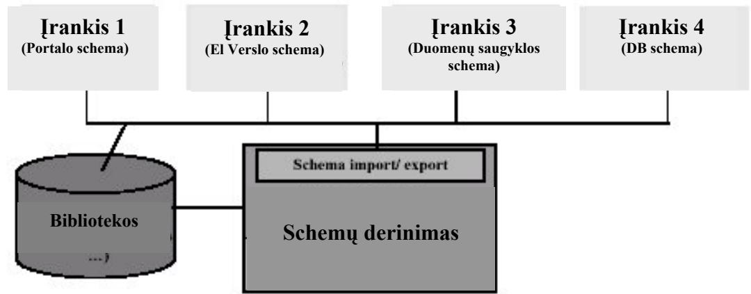
3.1 pav. Aukšto lygio architektūros derinimas
