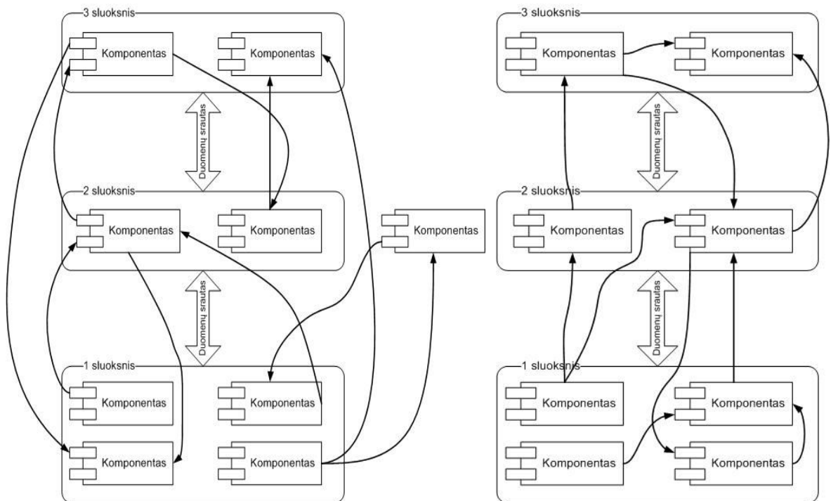
1 pav. Netaisyklingos(kairėje) ir taisyklingos(dešinėje) daugiasluoksnės architektūros pavyzdys.
