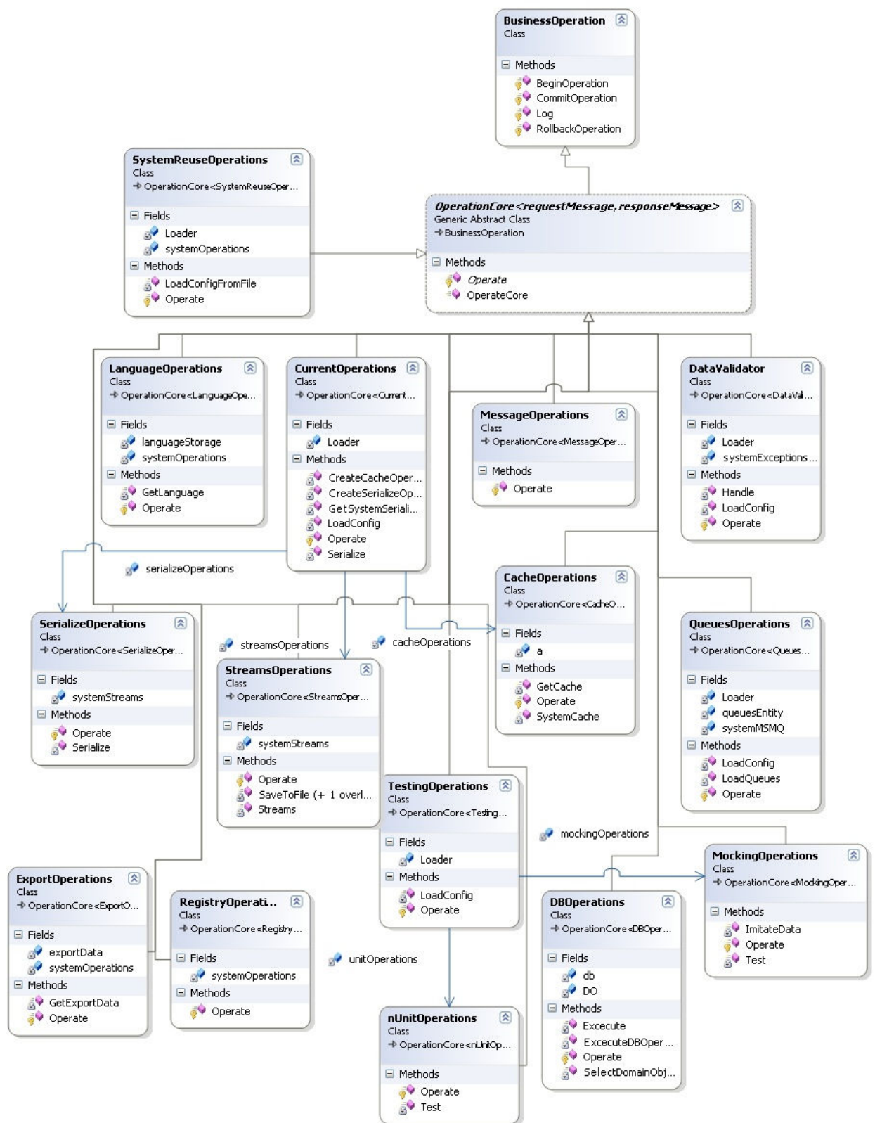
12 pav. Paketo „Operations“ klasių diagrama.
