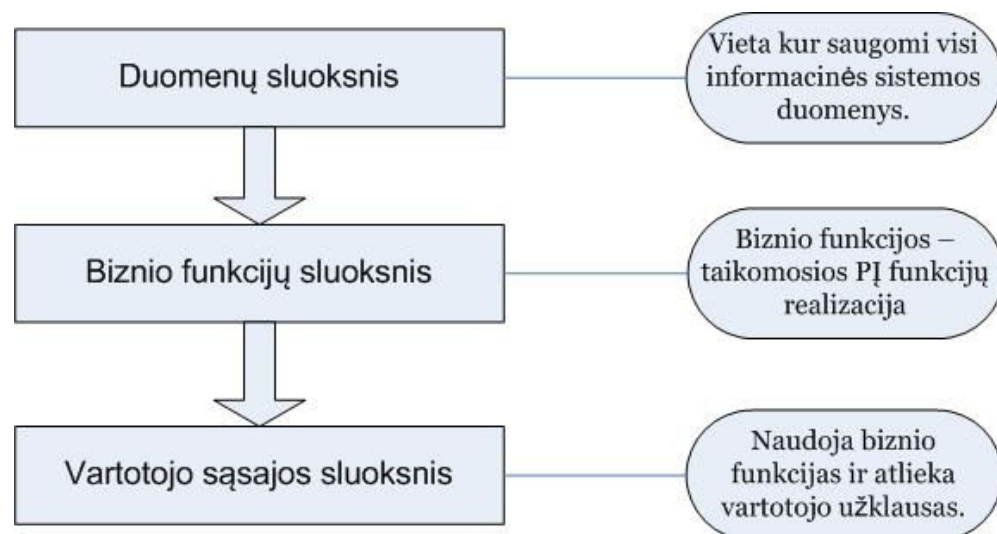
2 pav. Karkaso daugiasluoksnės architektūros diagrama.
