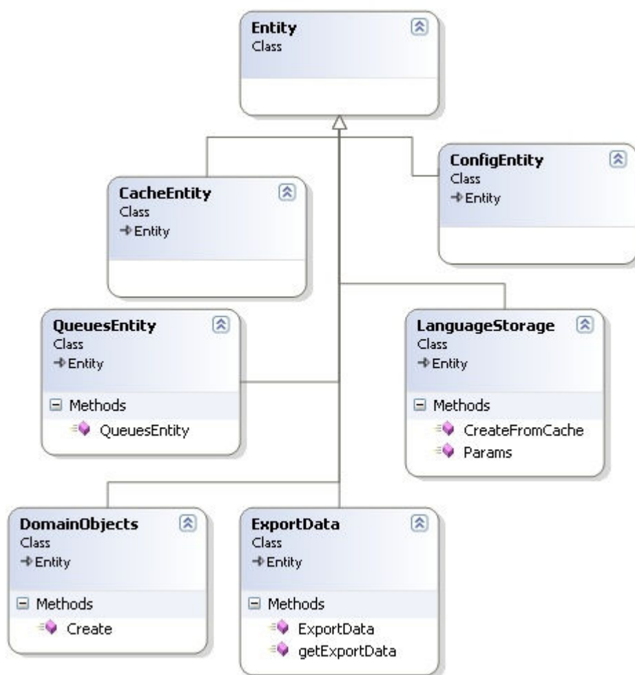
14 pav. Paketo „Entities“ klasių diagrama.
