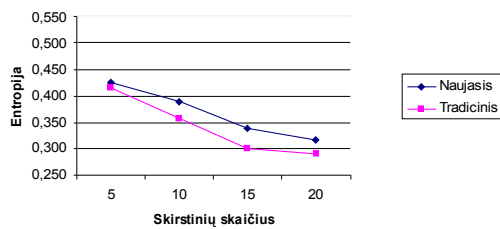
30 pav. Metodų entropijos įvertinimas klasterizuojant 8448 dokumentų kolekciją
