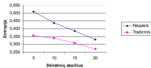
26 pav. Metodų entropijos įvertinimas klasterizuojant 2112 dokumentų kolekciją
