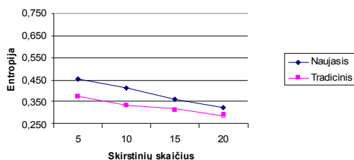
32 pav. Metodų klasterizavimo entropijos vidurkiai
