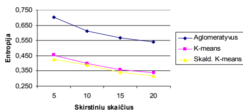
20 pav. 8448 dokumentų kolekcijos klasterizavimo entropijos įvertinimai
